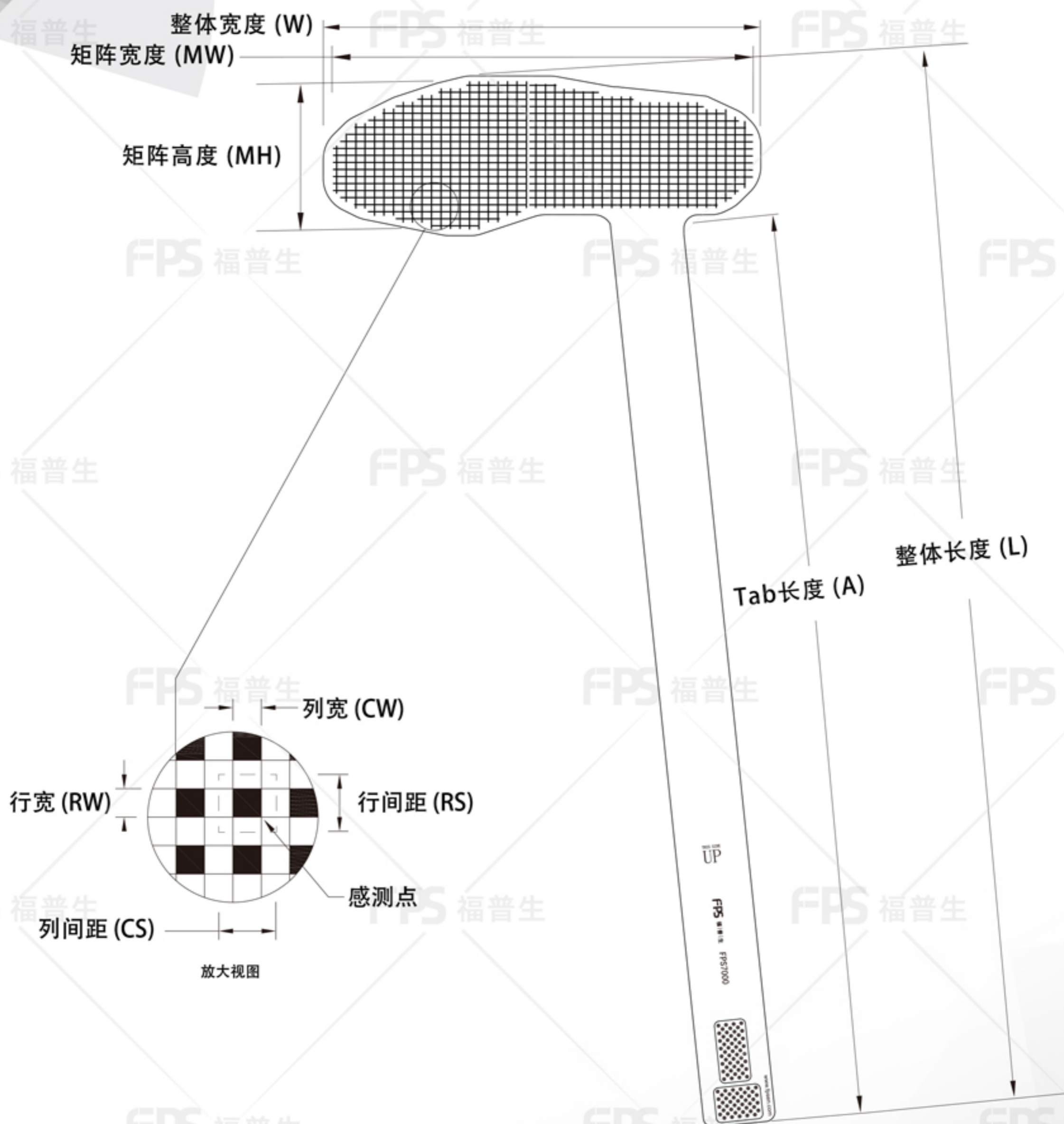
外形尺寸
