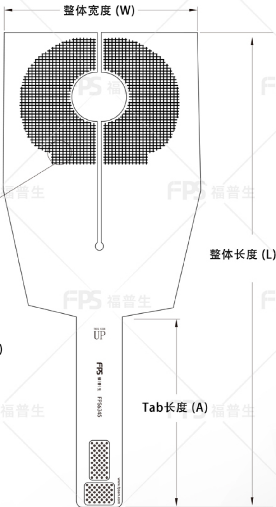
传感区参数
