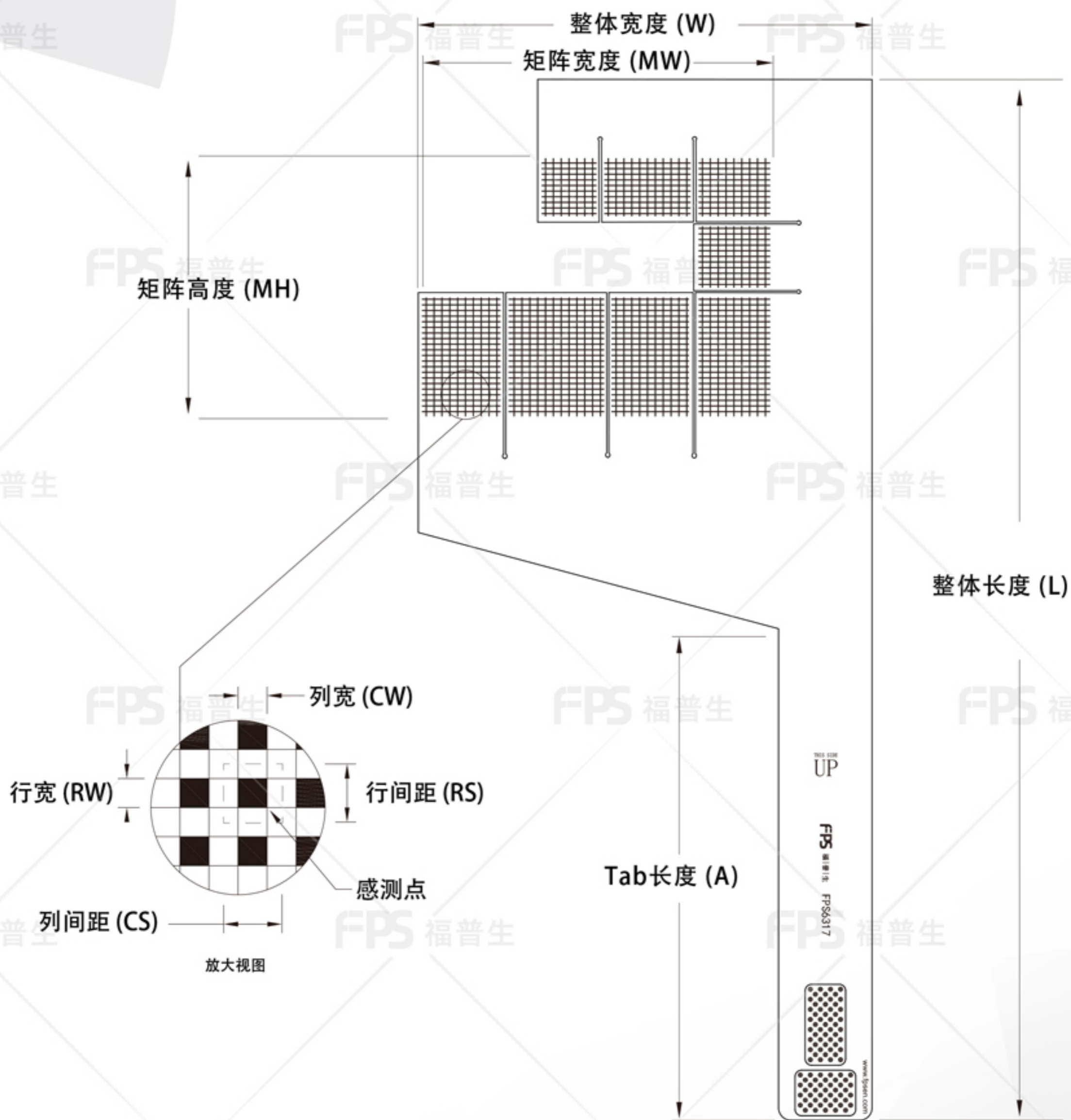
外形尺寸
