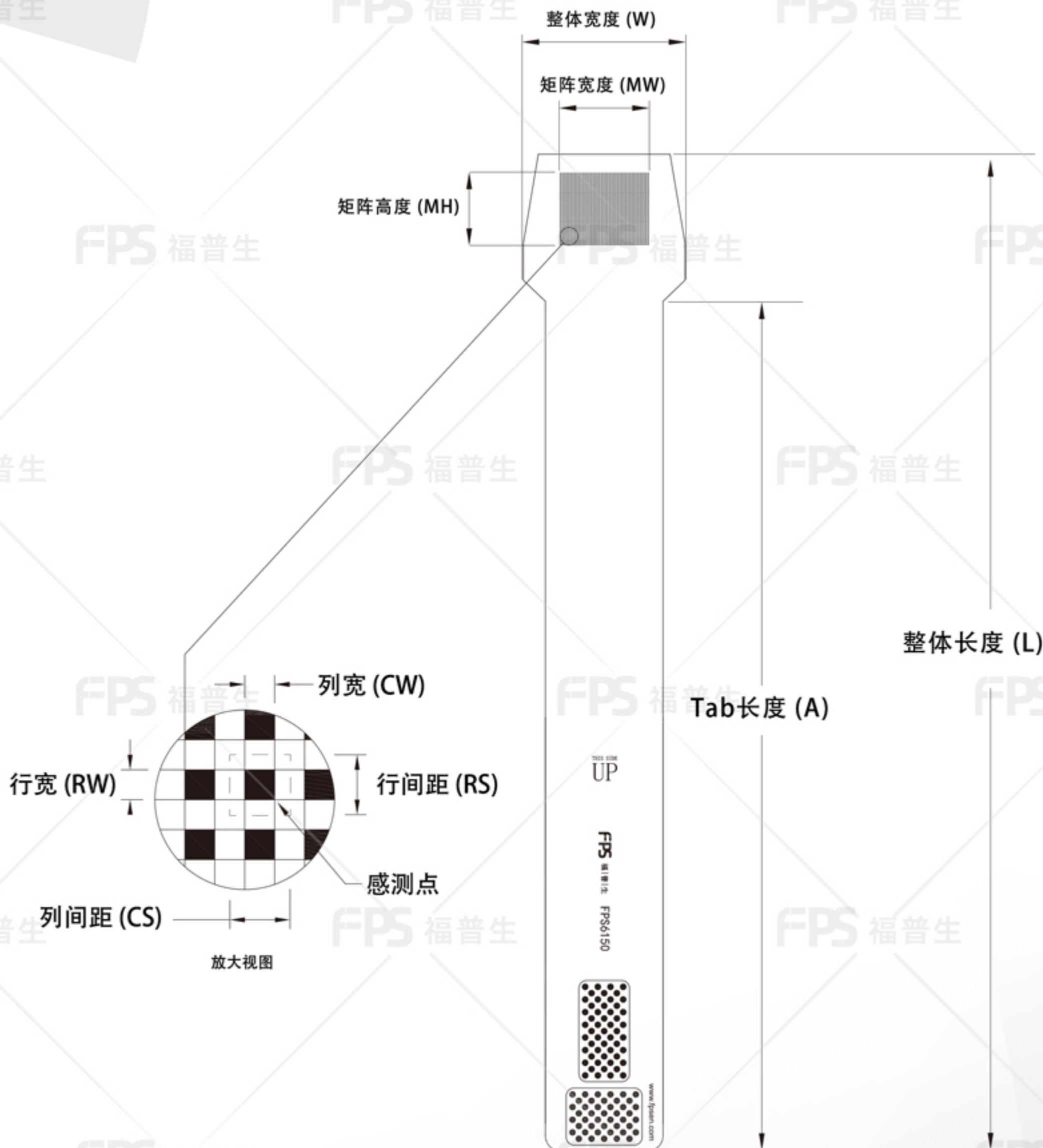
外形尺寸
