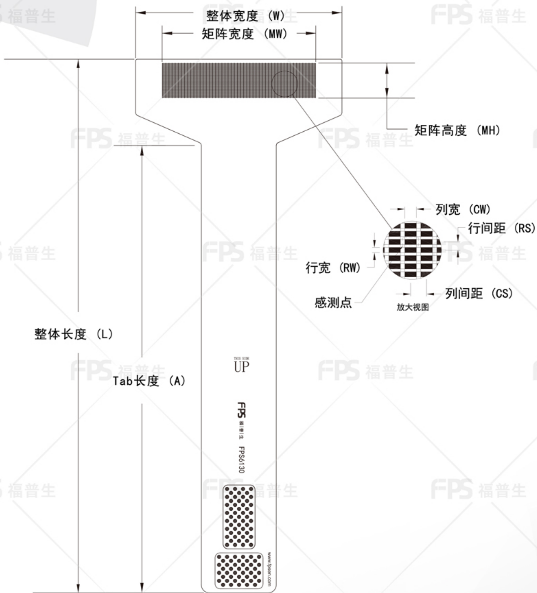
外形尺寸
