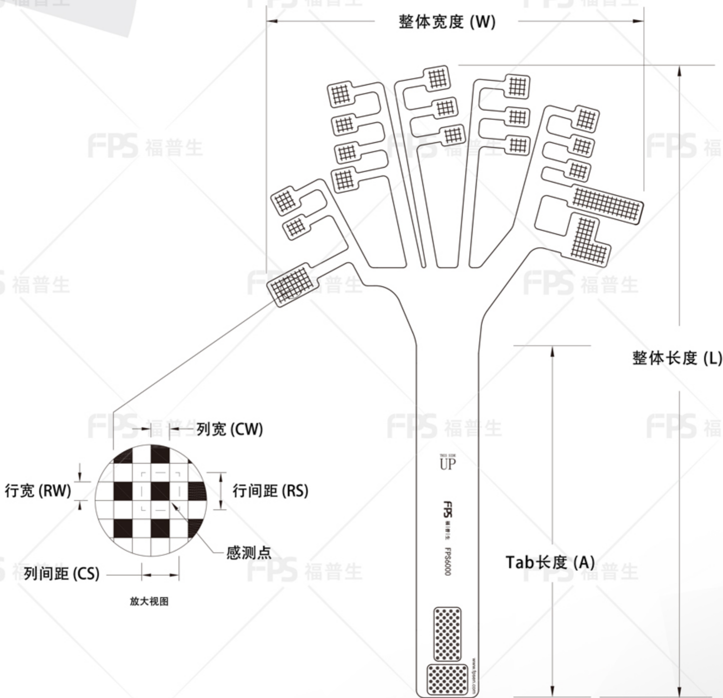
外形尺寸
