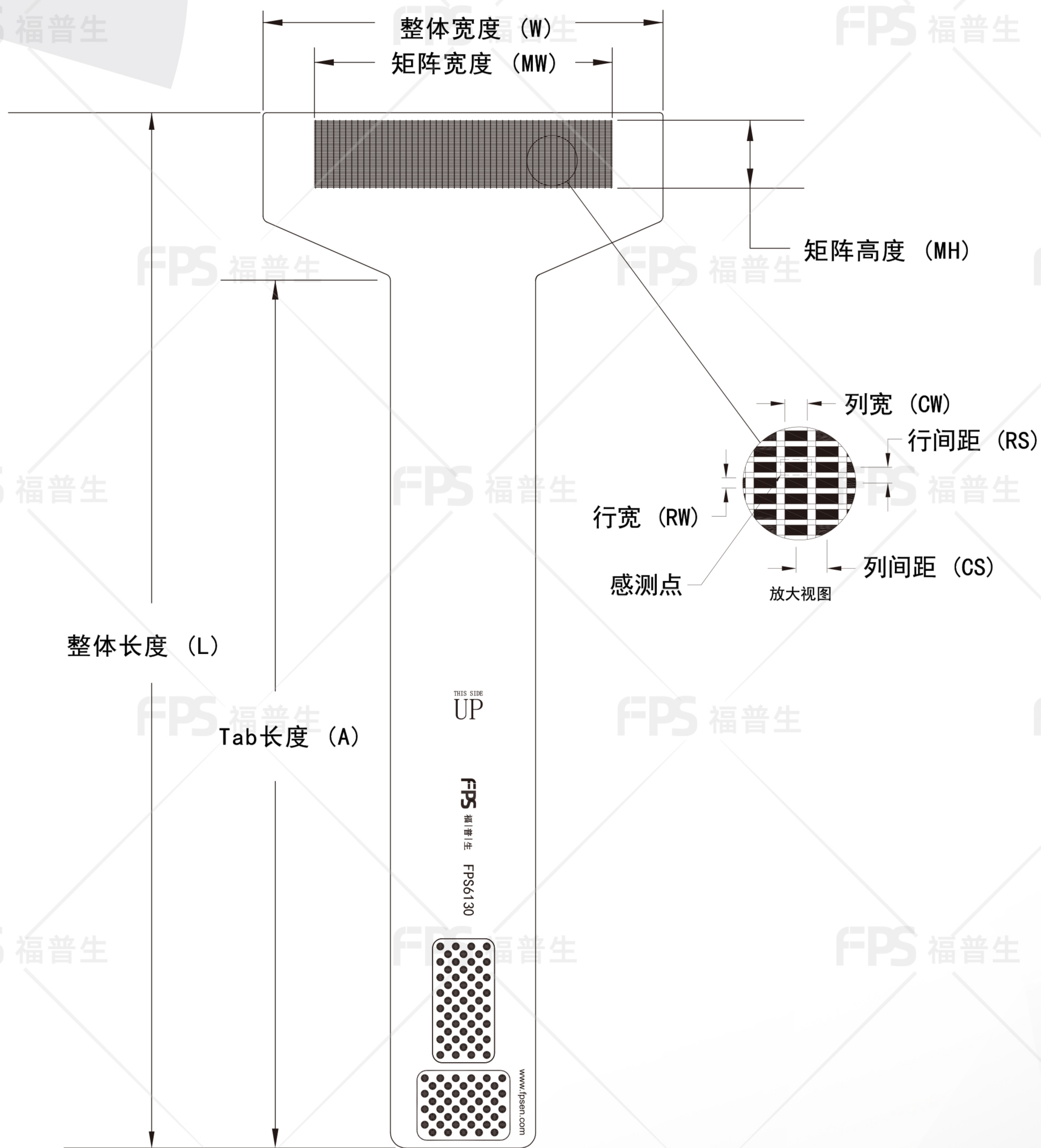
外形尺寸
