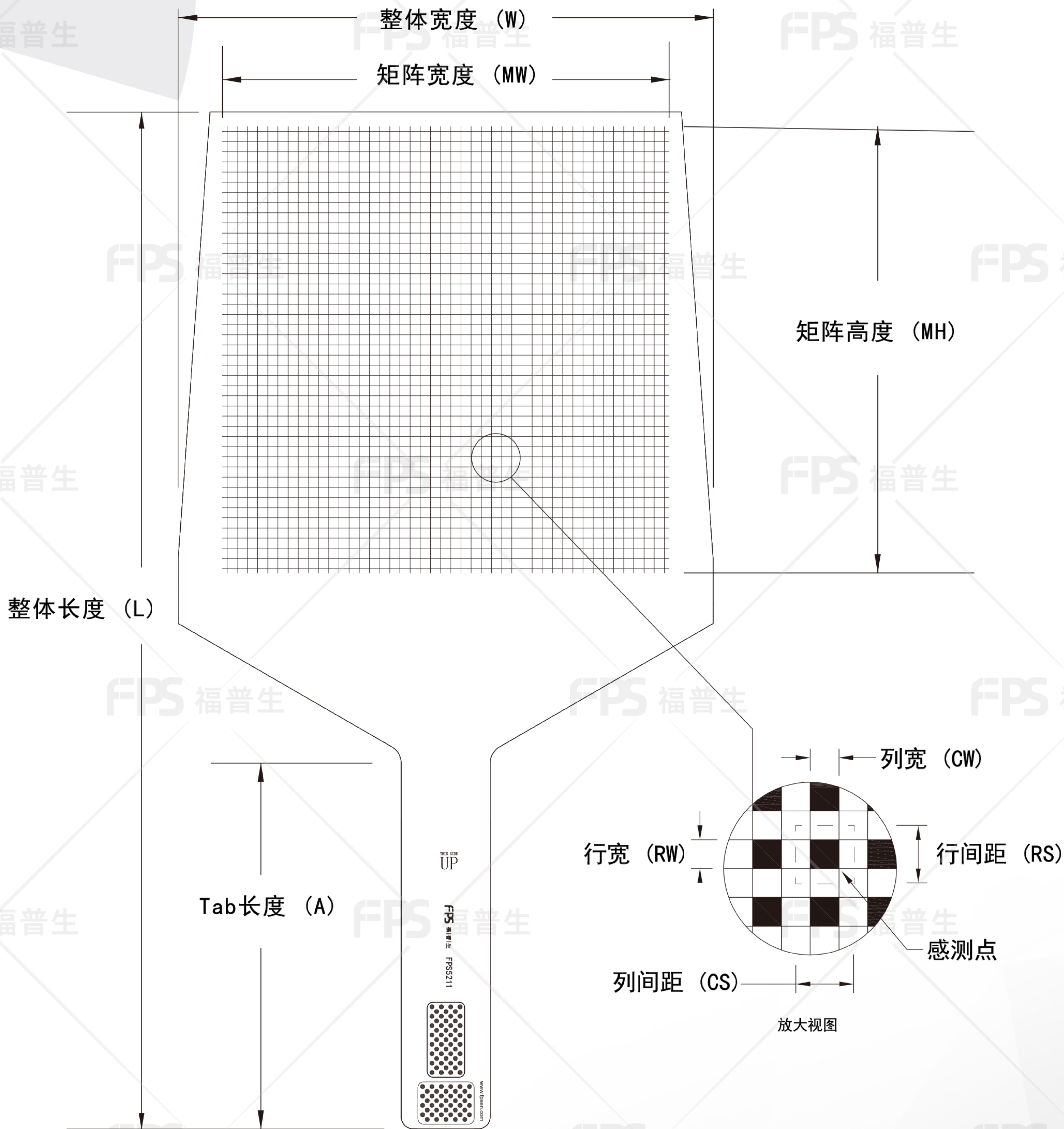
外形尺寸
