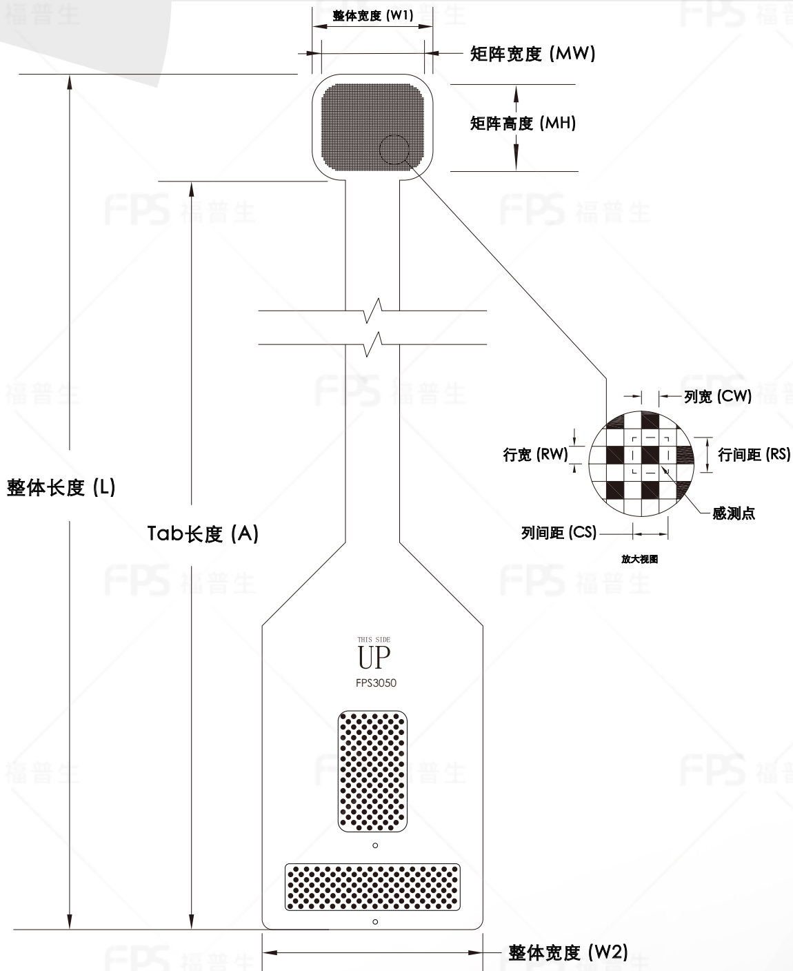
外形尺寸
