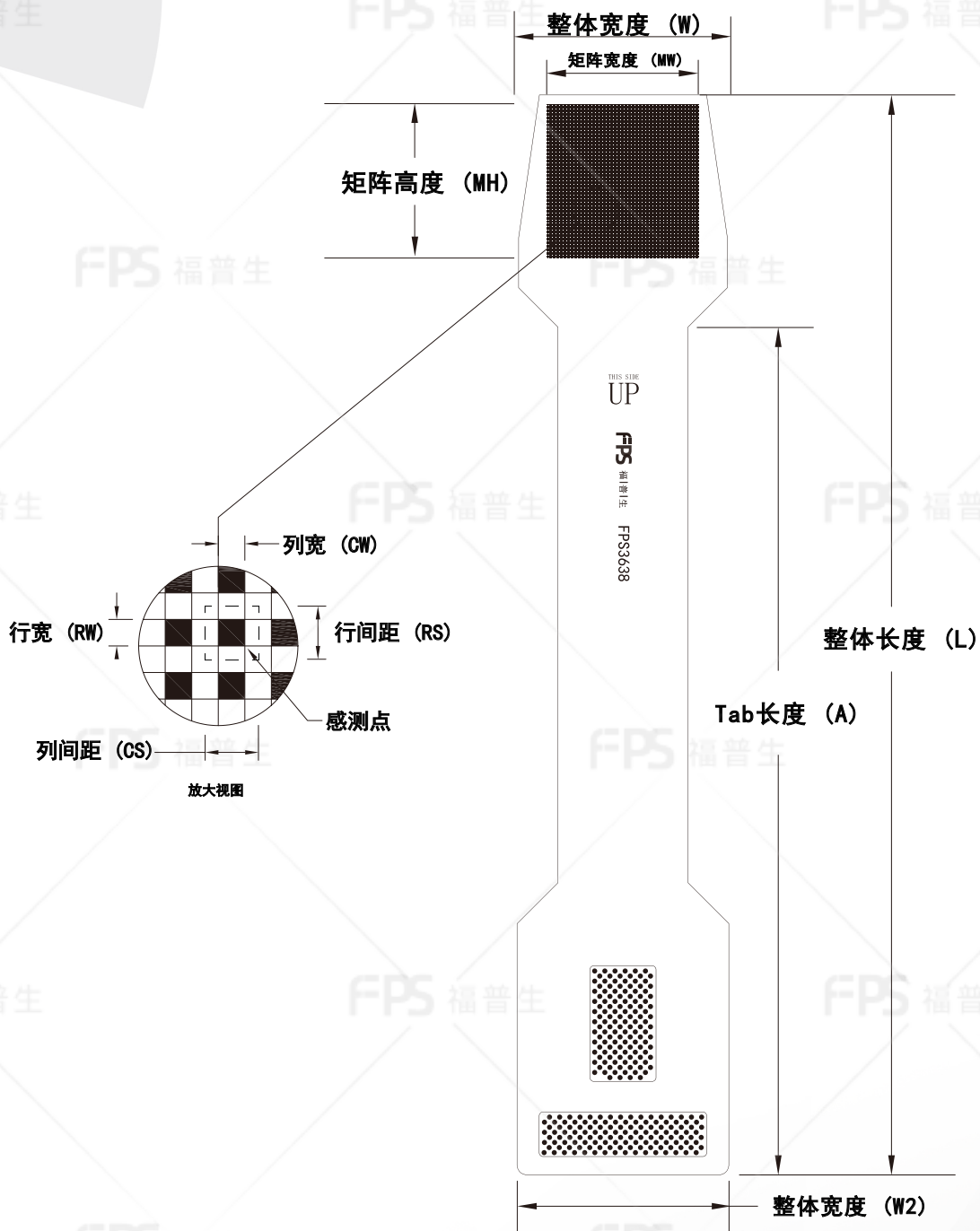
外形尺寸
