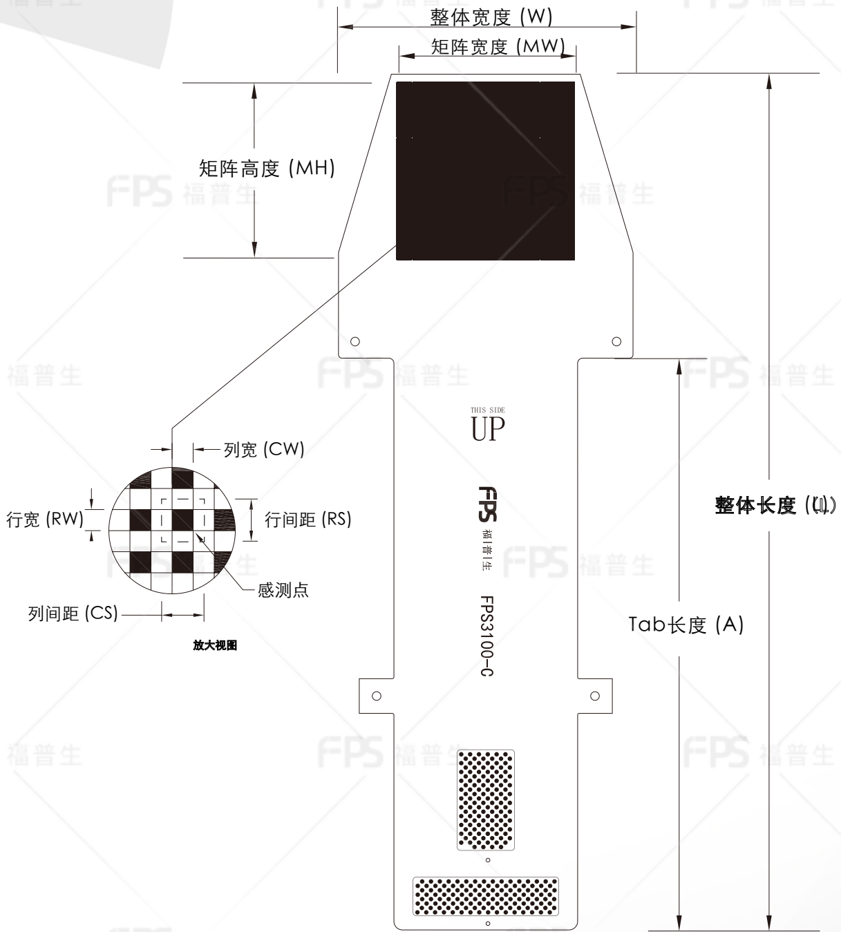
外形尺寸
