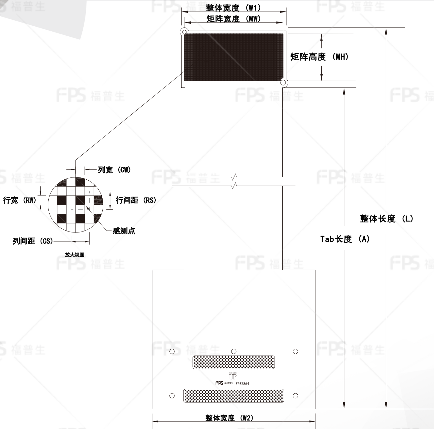
外形尺寸
