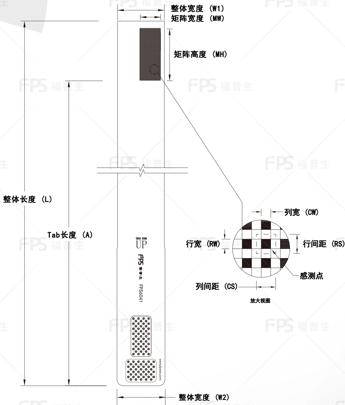
外形尺寸
