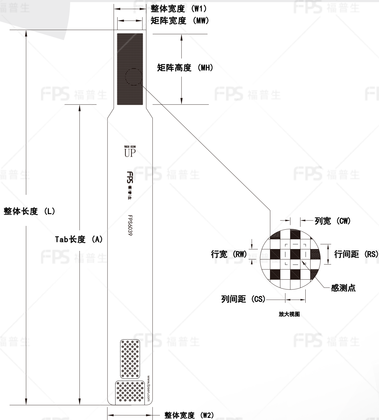
外形尺寸
