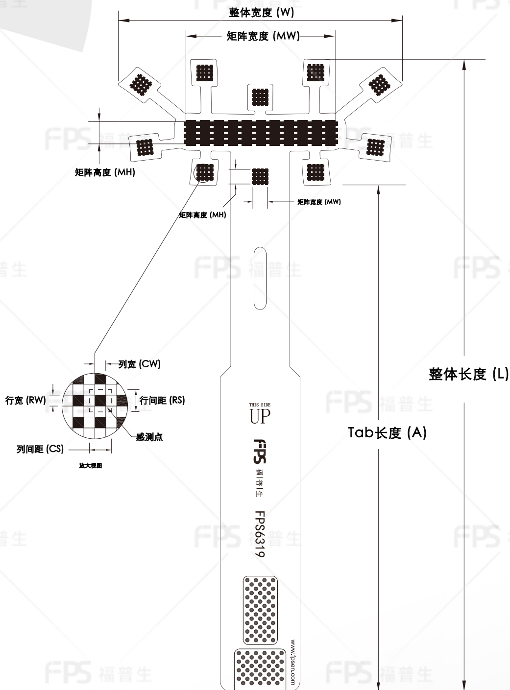
外形尺寸
