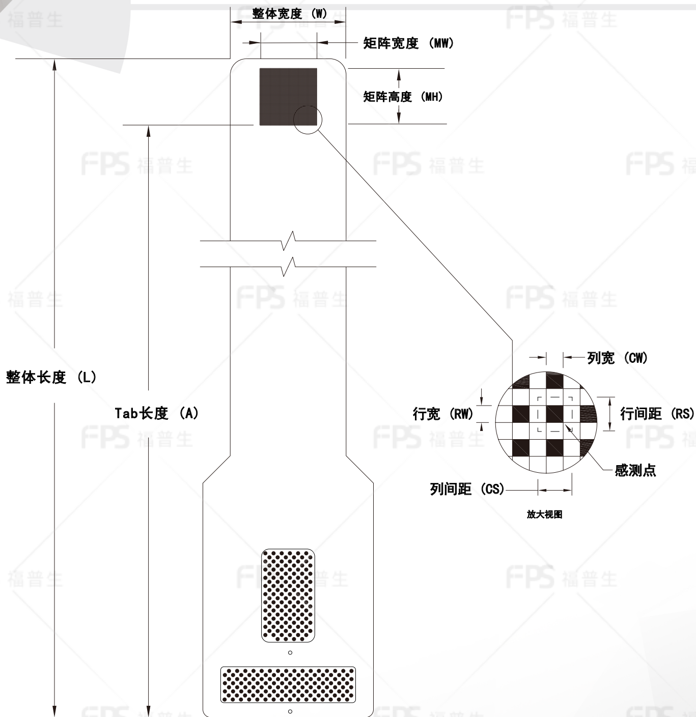
外形尺寸
