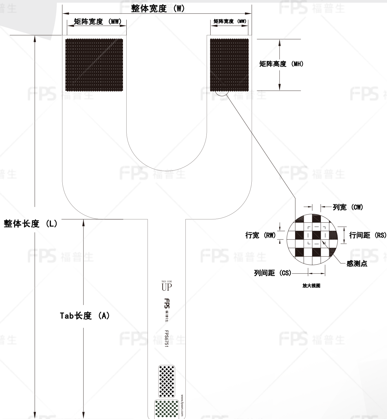
外形尺寸
