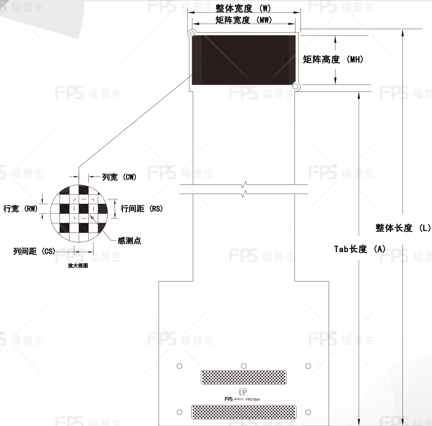
外形尺寸
