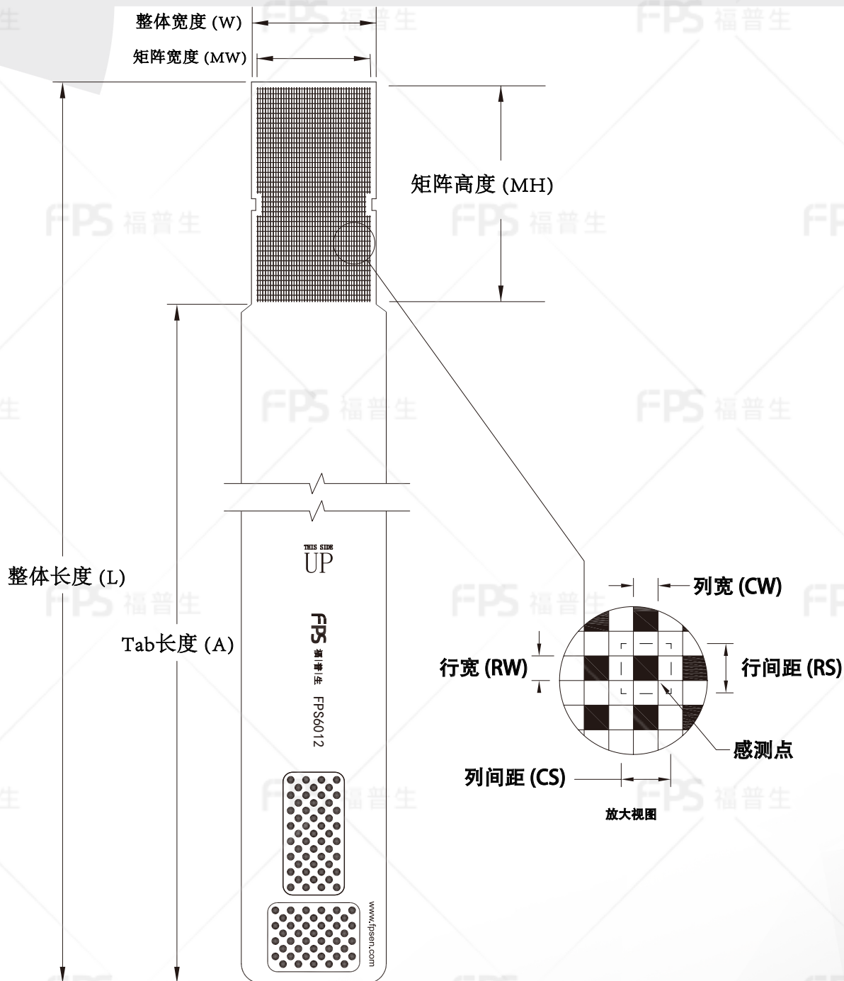
外形尺寸
