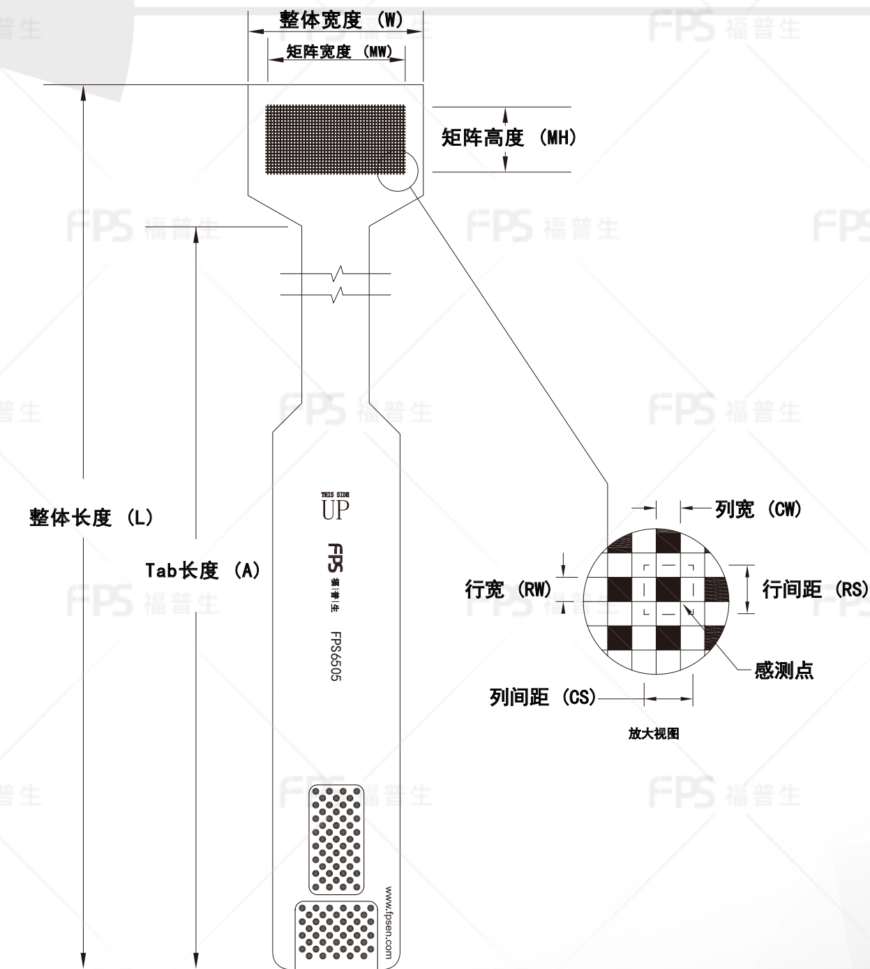
外形尺寸
