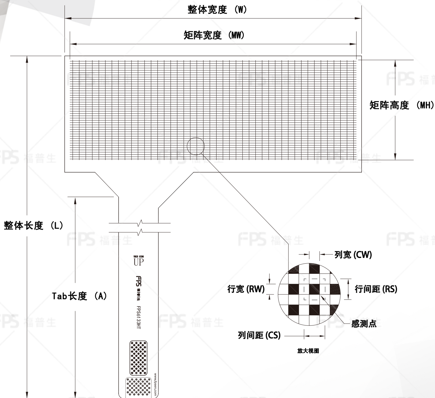
外形尺寸
