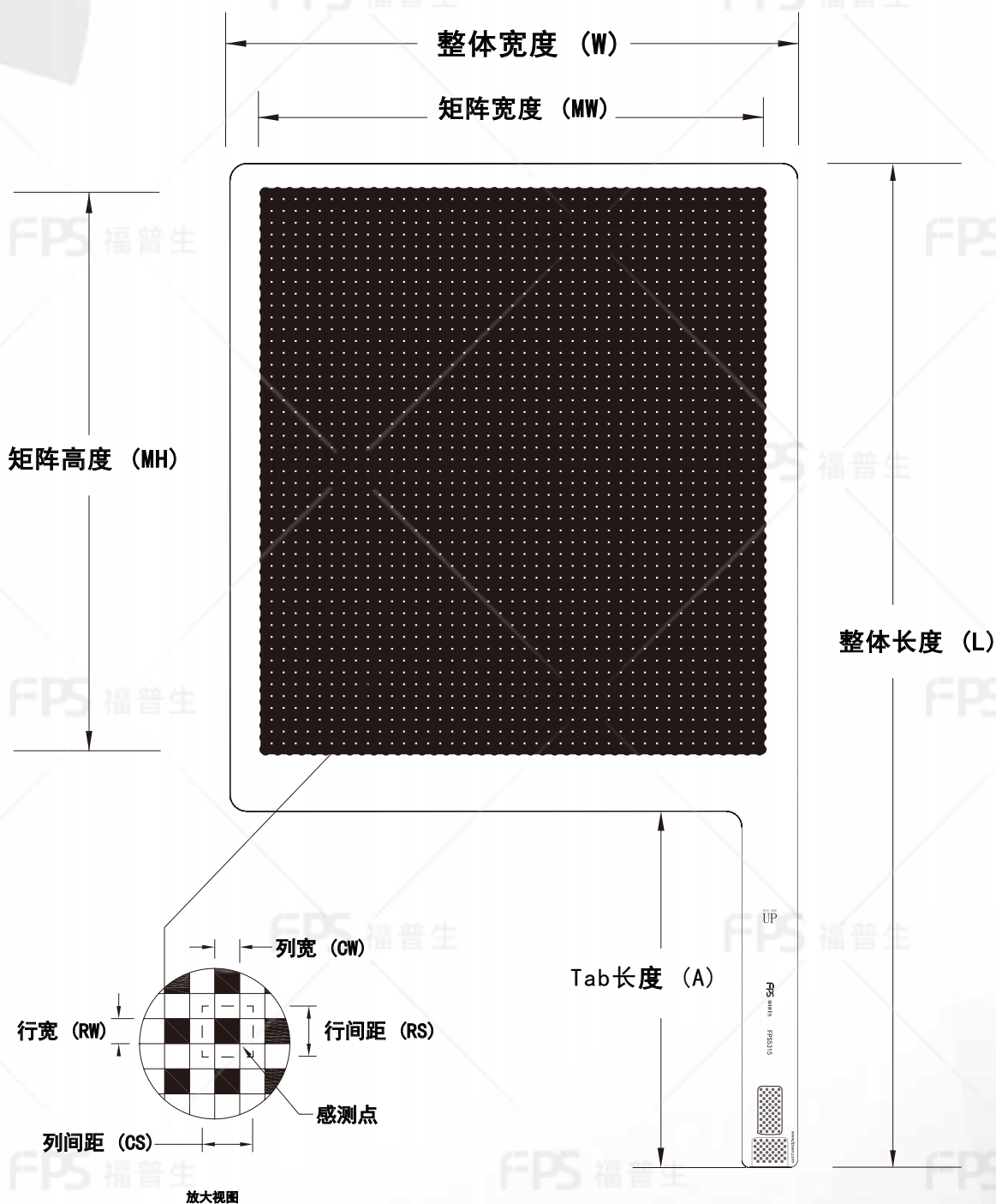
传感区参数
