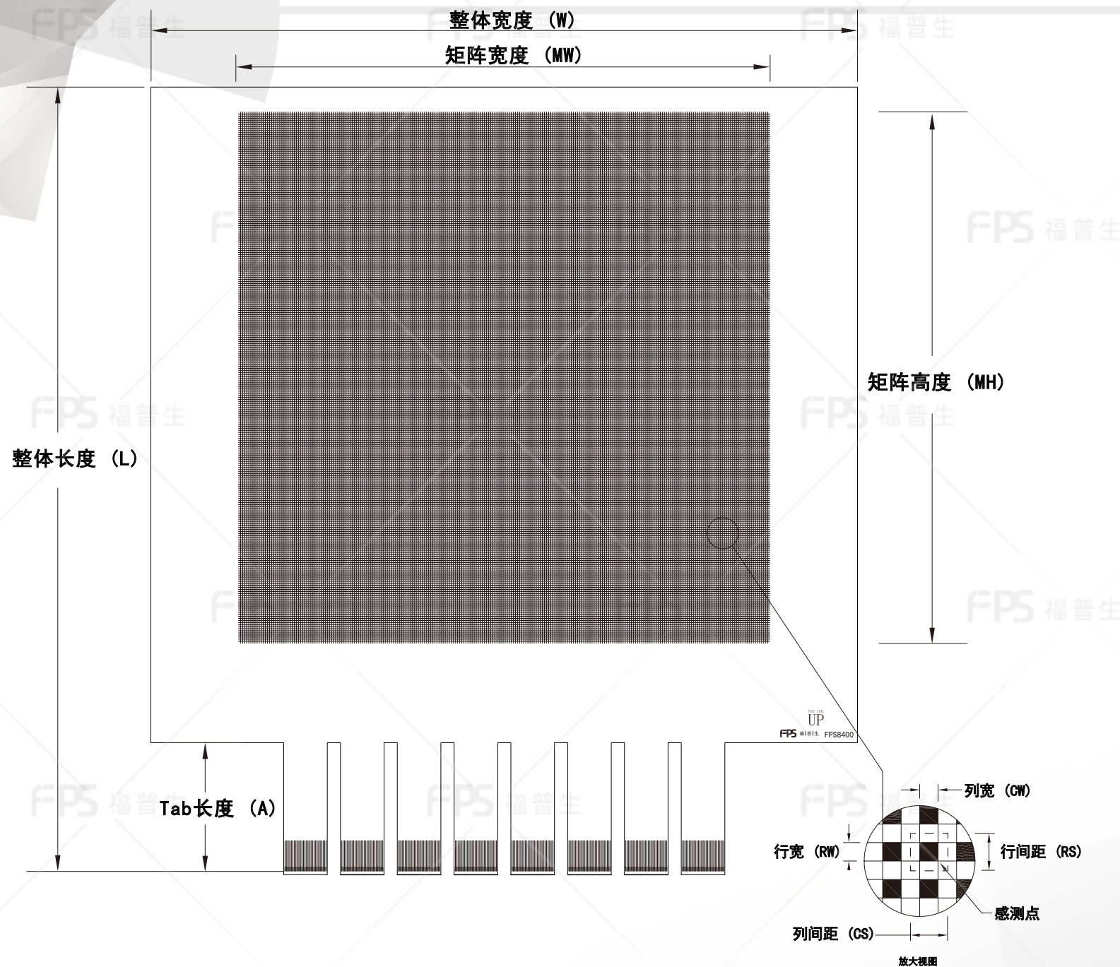
外形尺寸
