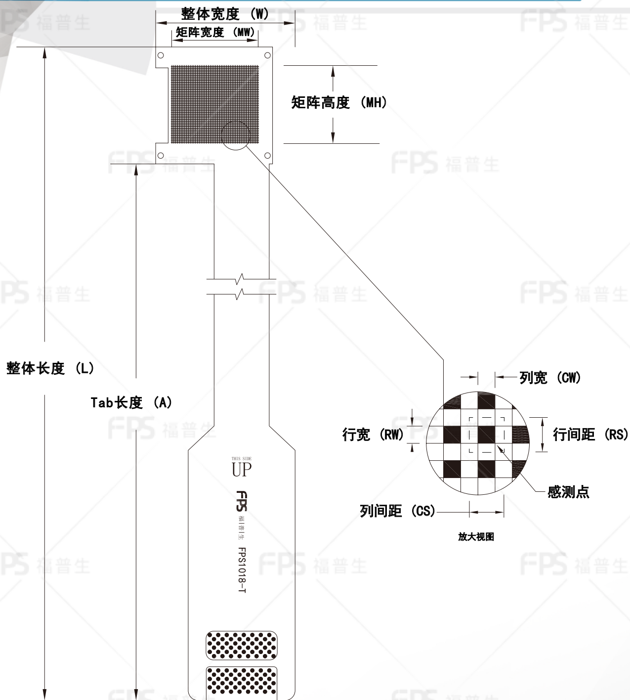
外形尺寸
