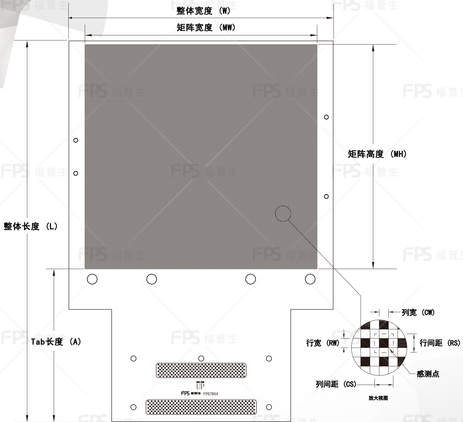
外形尺寸
