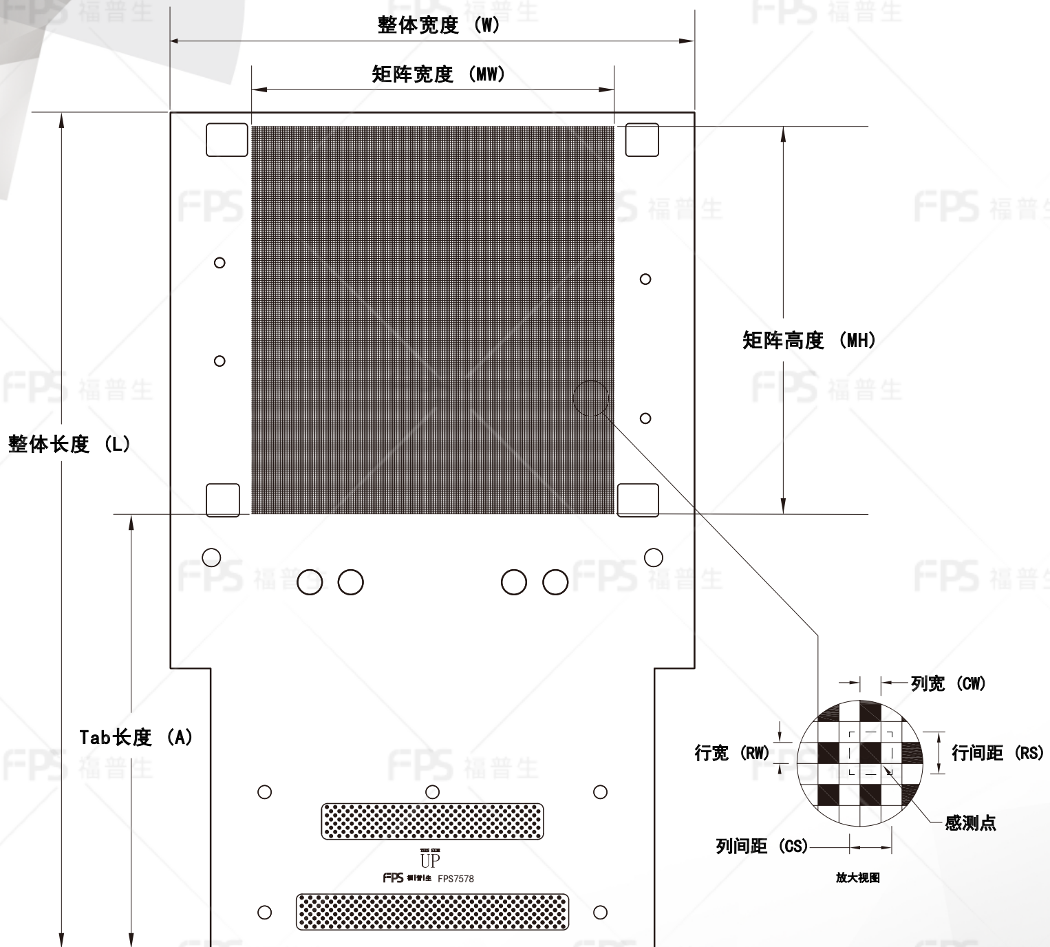
外形尺寸
