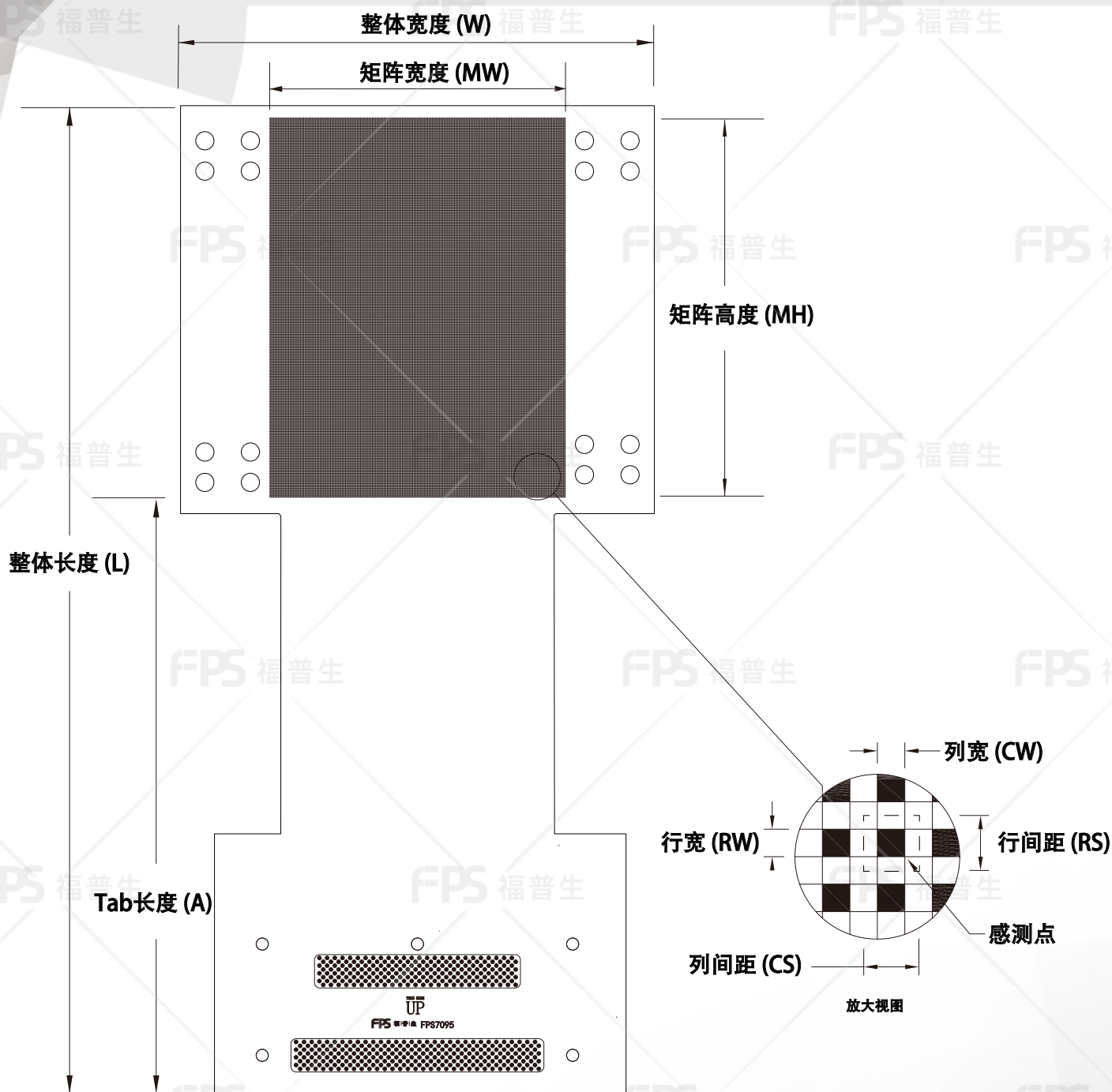
外形尺寸
