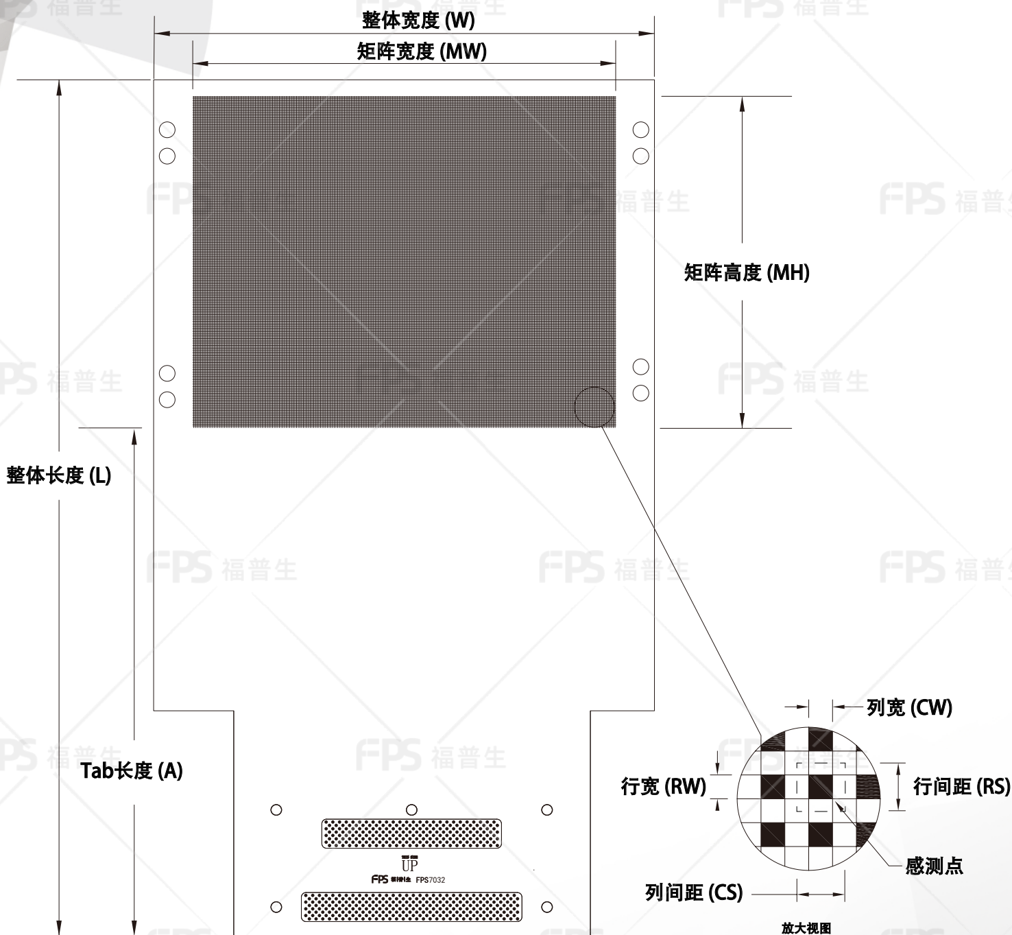
外形尺寸
