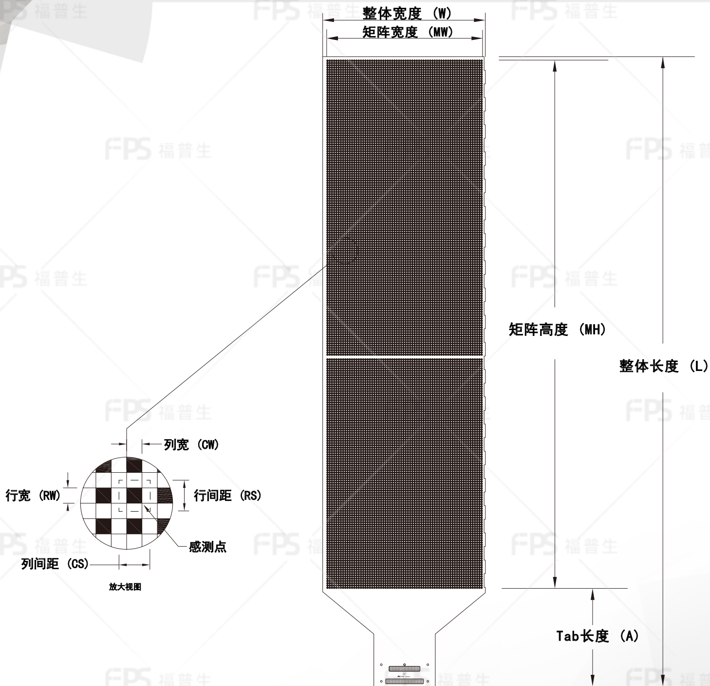
外形尺寸
