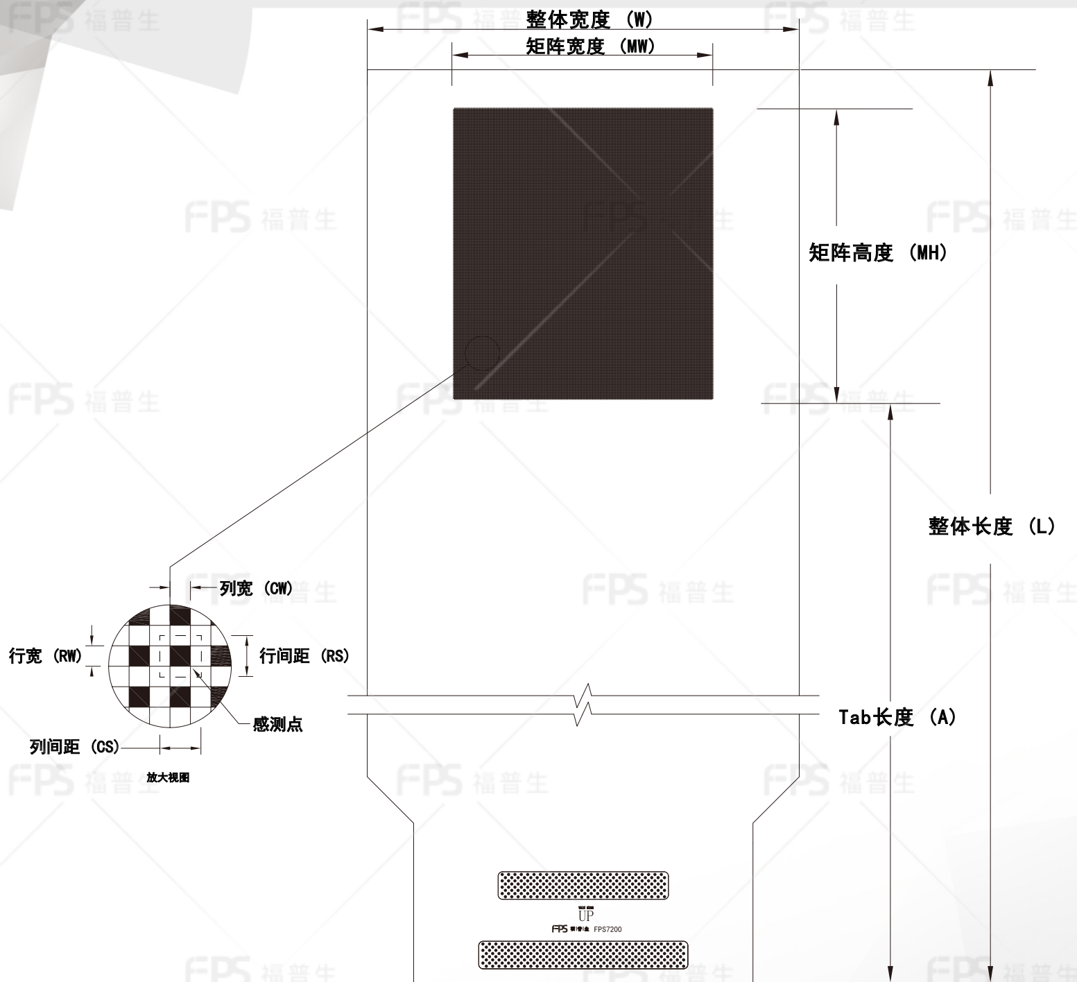
外形尺寸
