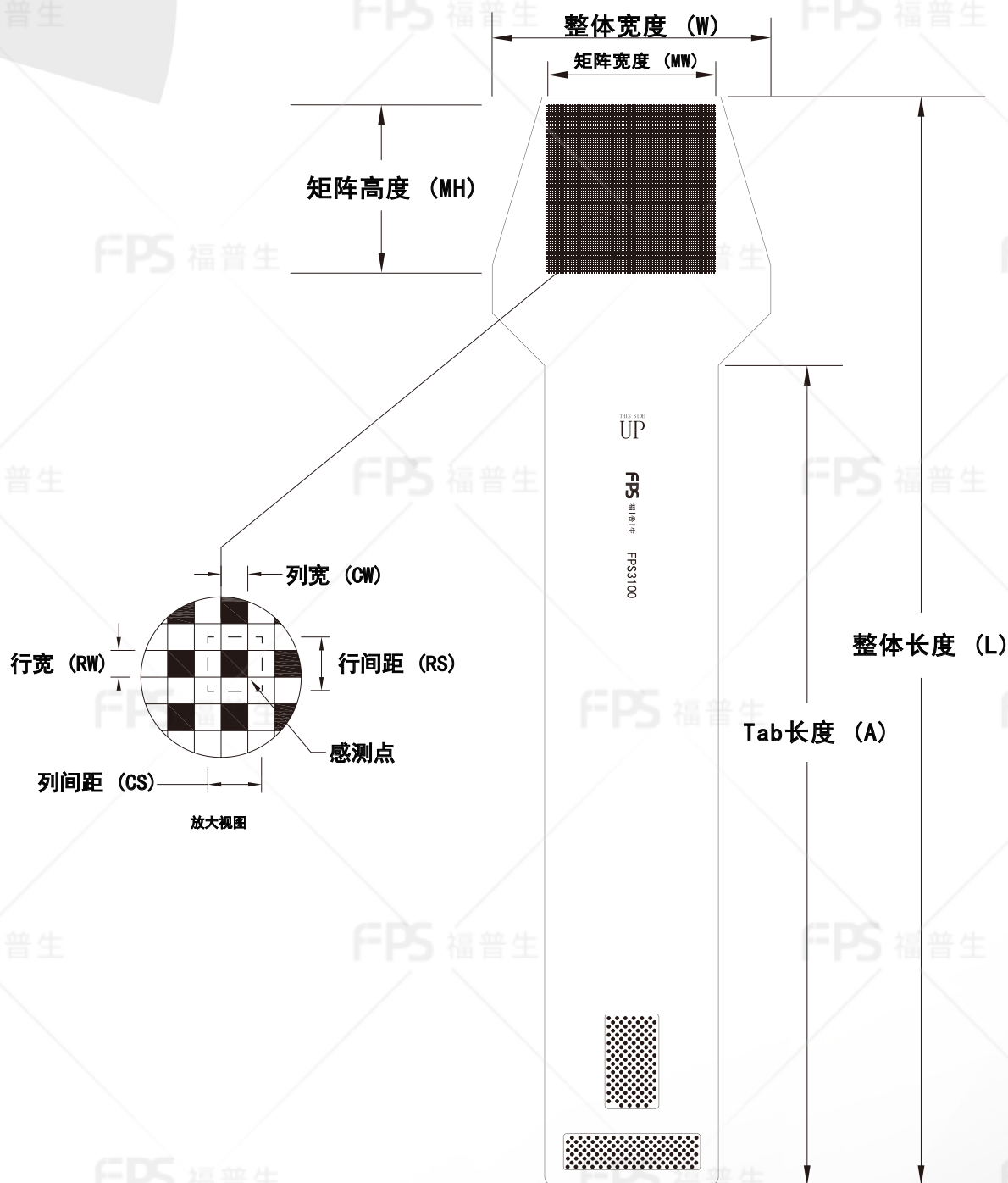
外形尺寸
