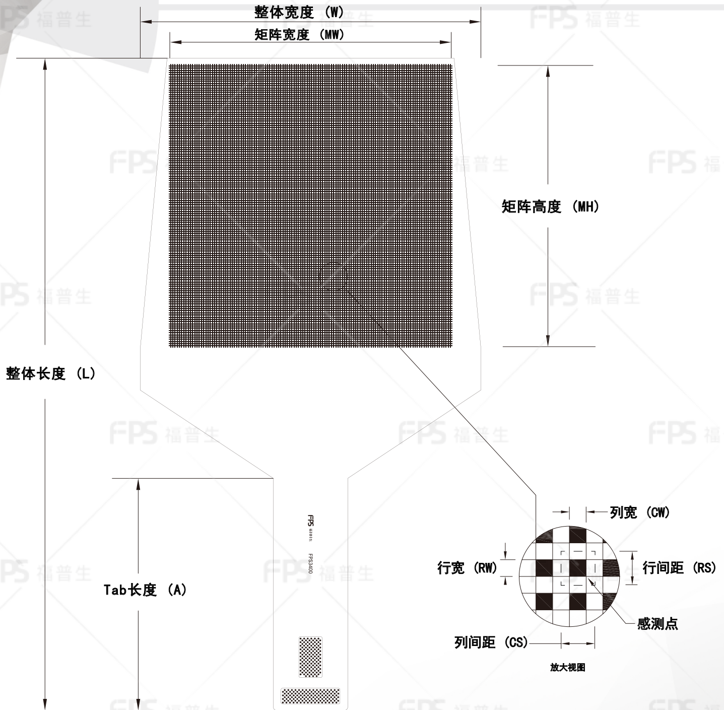
外形尺寸
