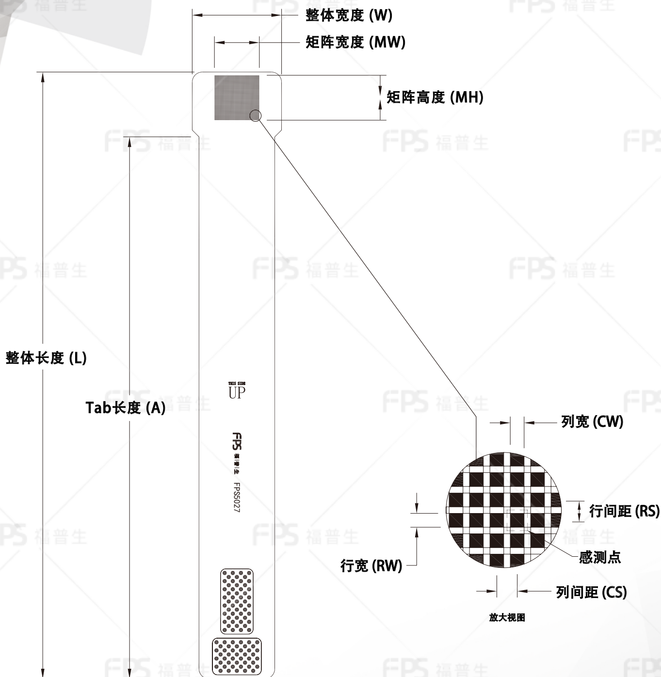
外形尺寸
