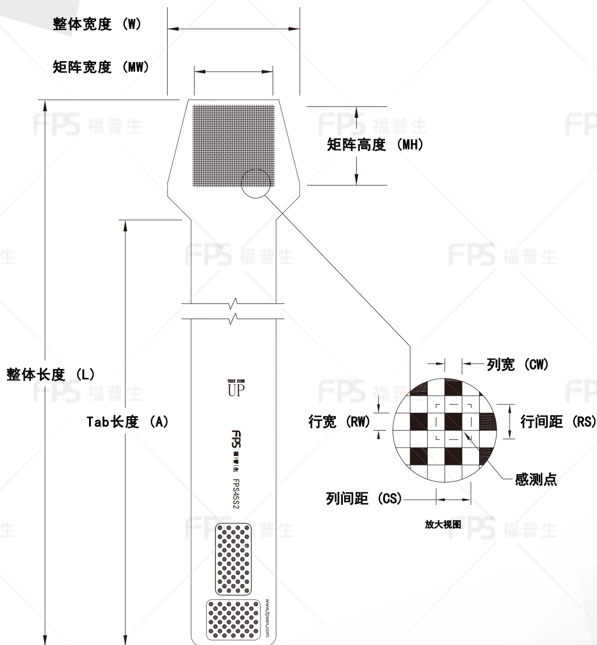
外形尺寸
