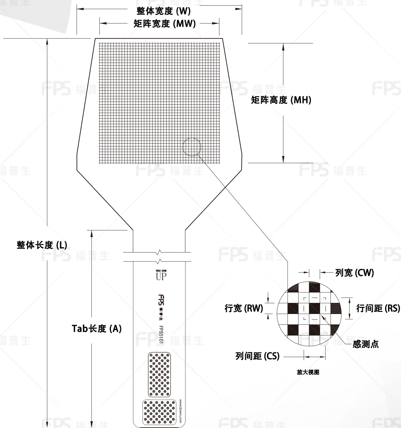
外形尺寸
