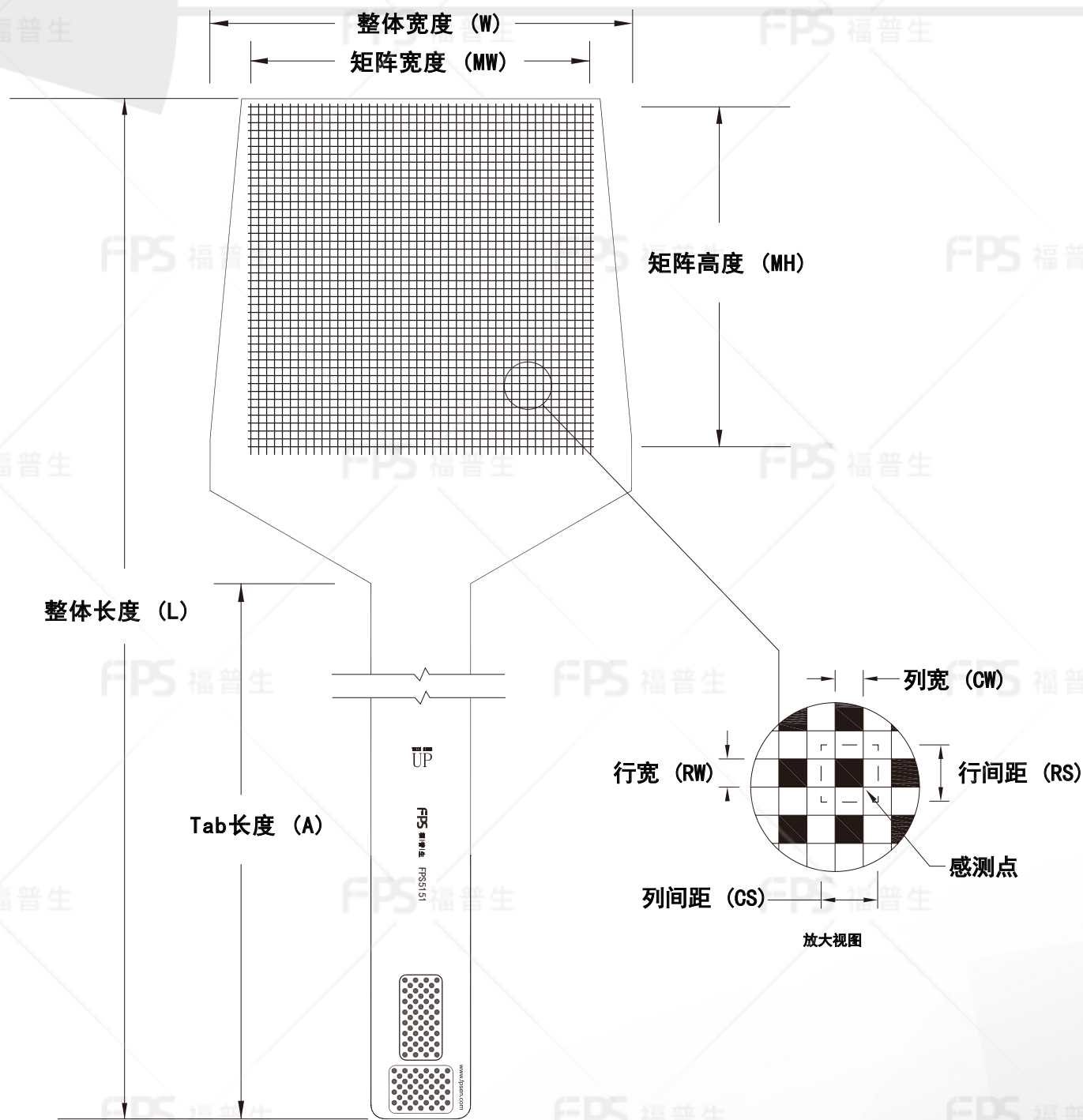
外形尺寸
