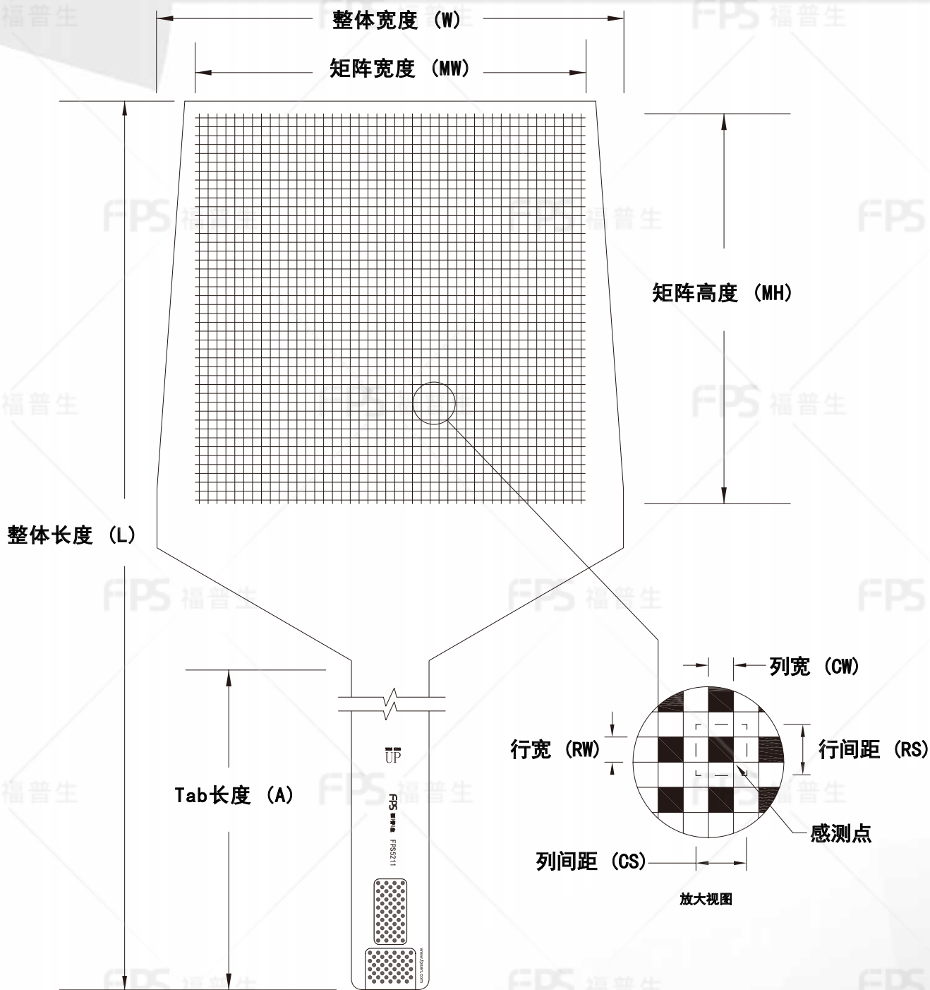
外形尺寸
