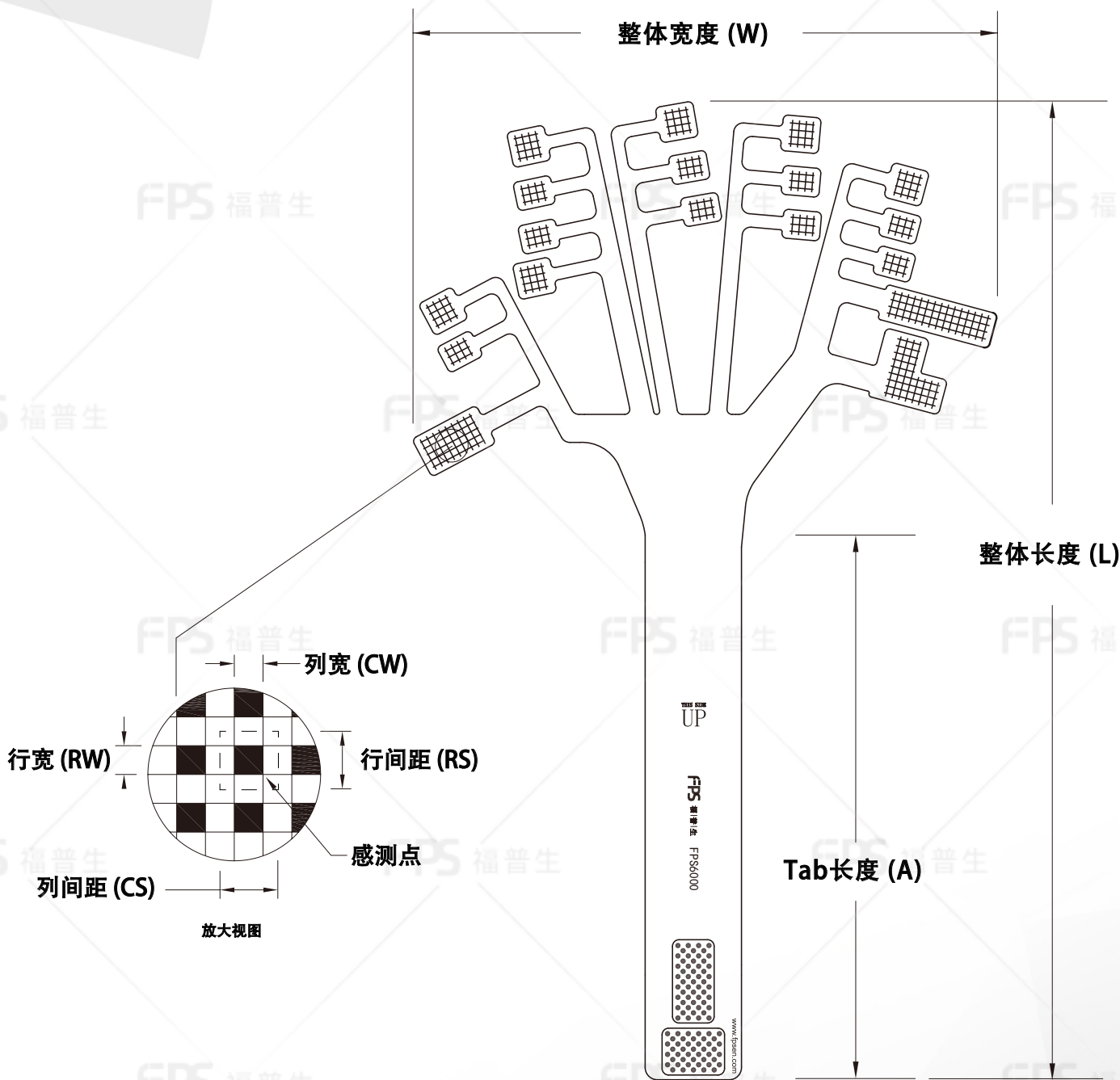
外形尺寸
