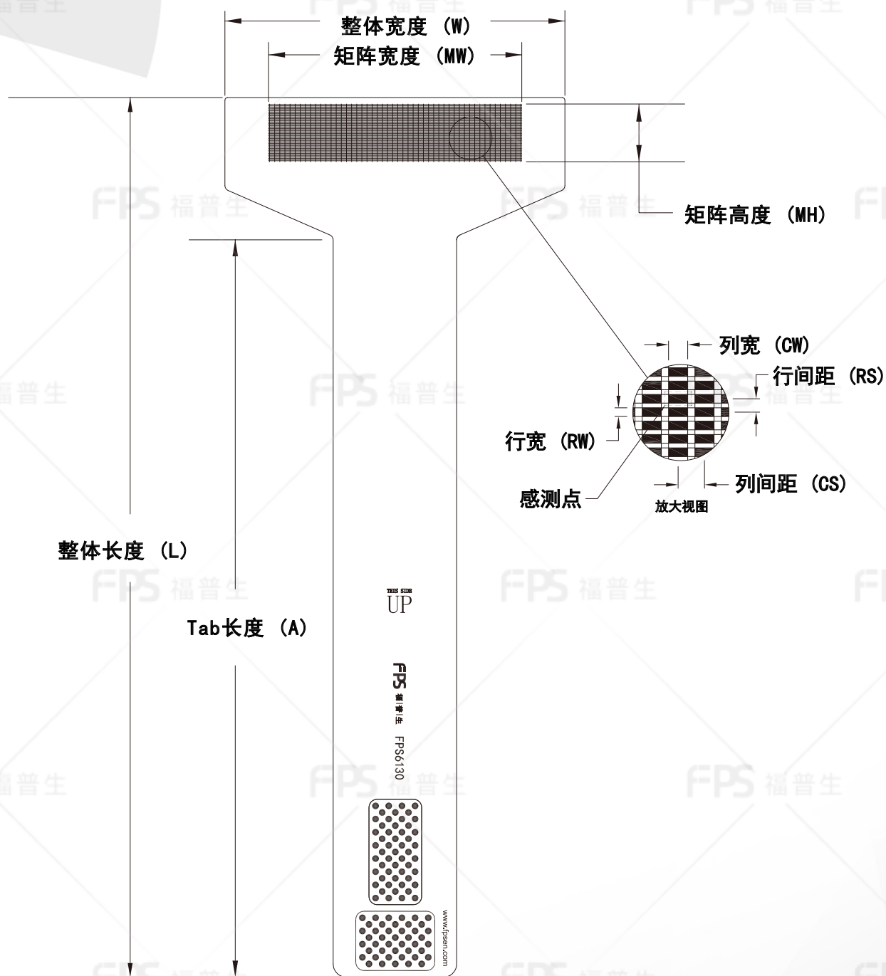
外形尺寸
