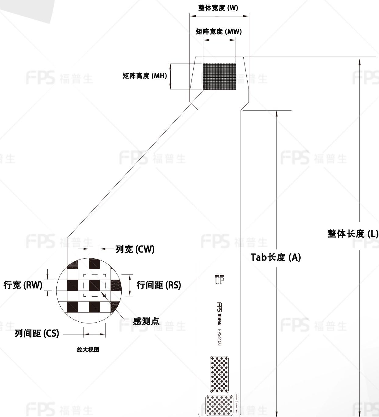
外形尺寸
