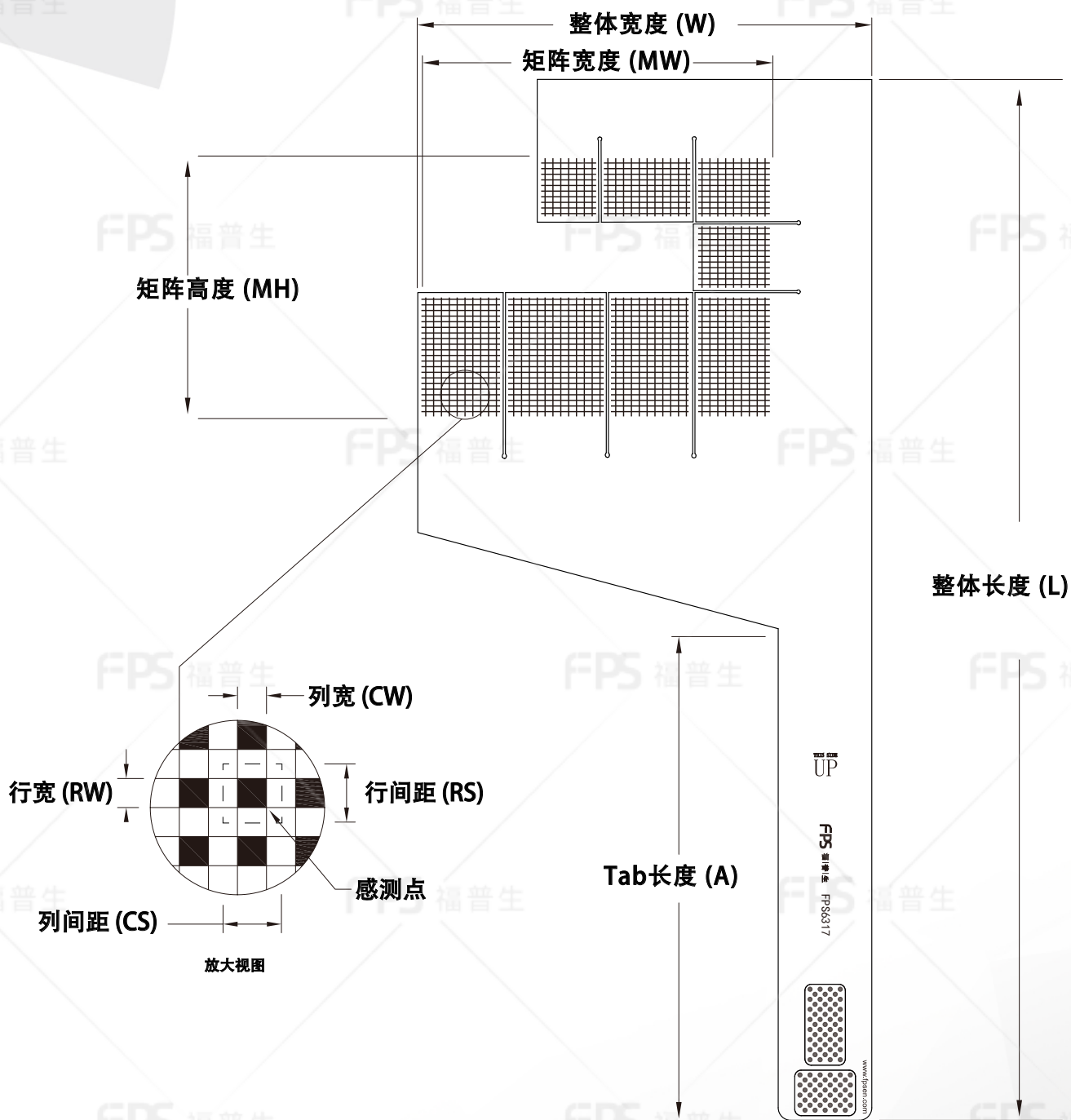
外形尺寸
