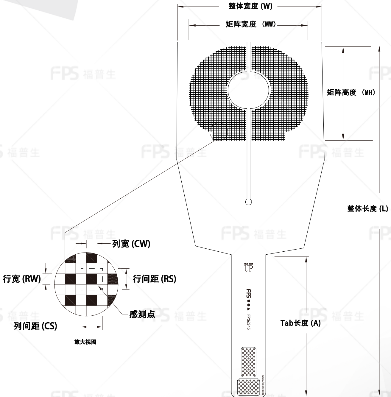
外形尺寸
