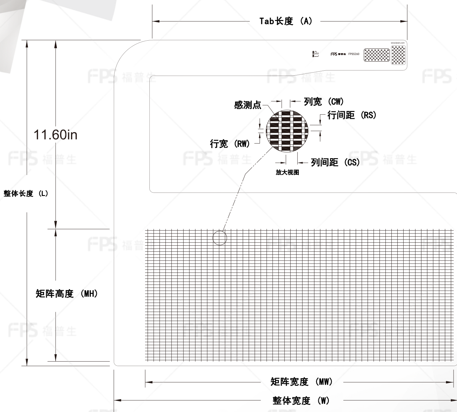
外形尺寸
