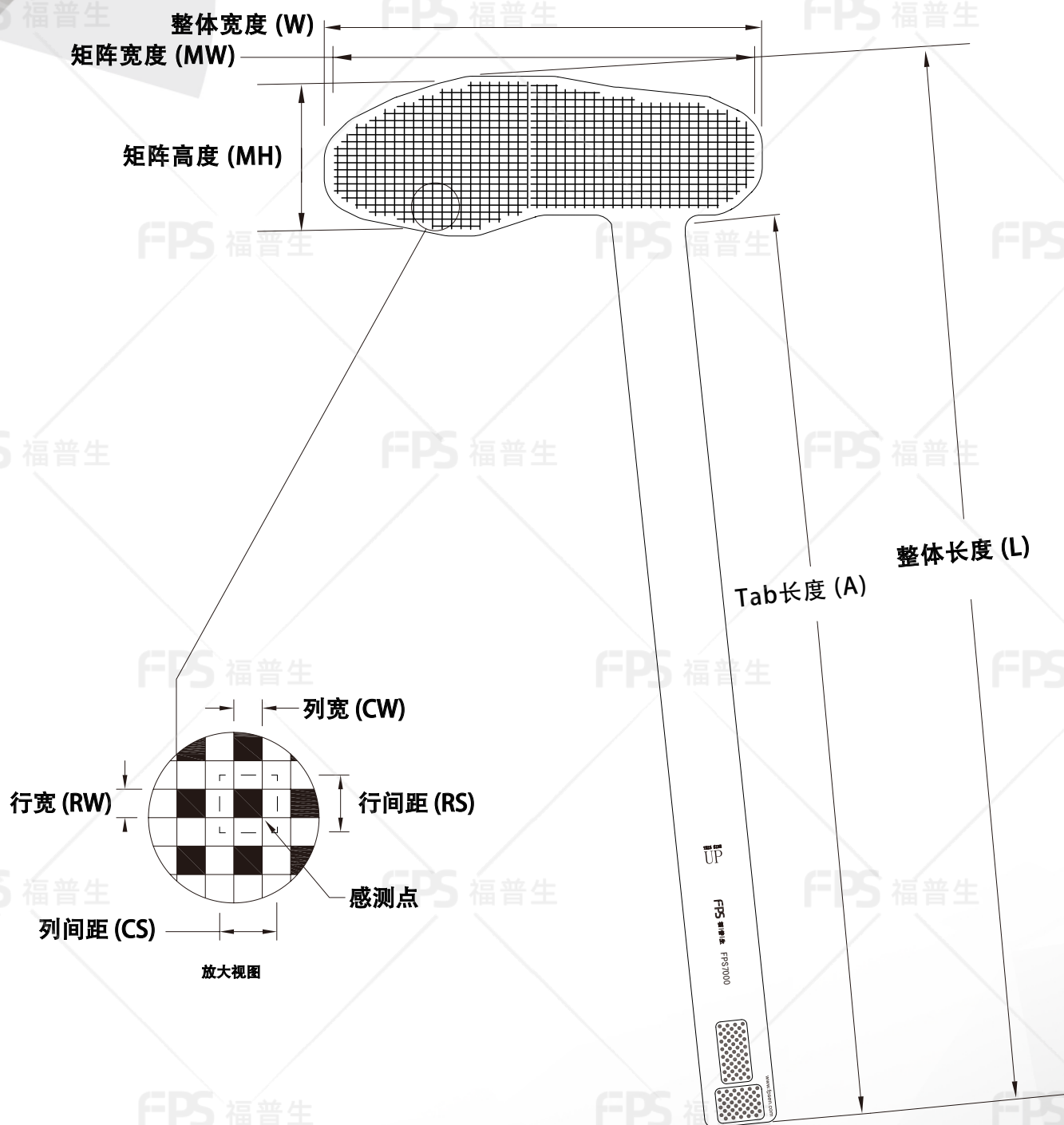
外形尺寸
