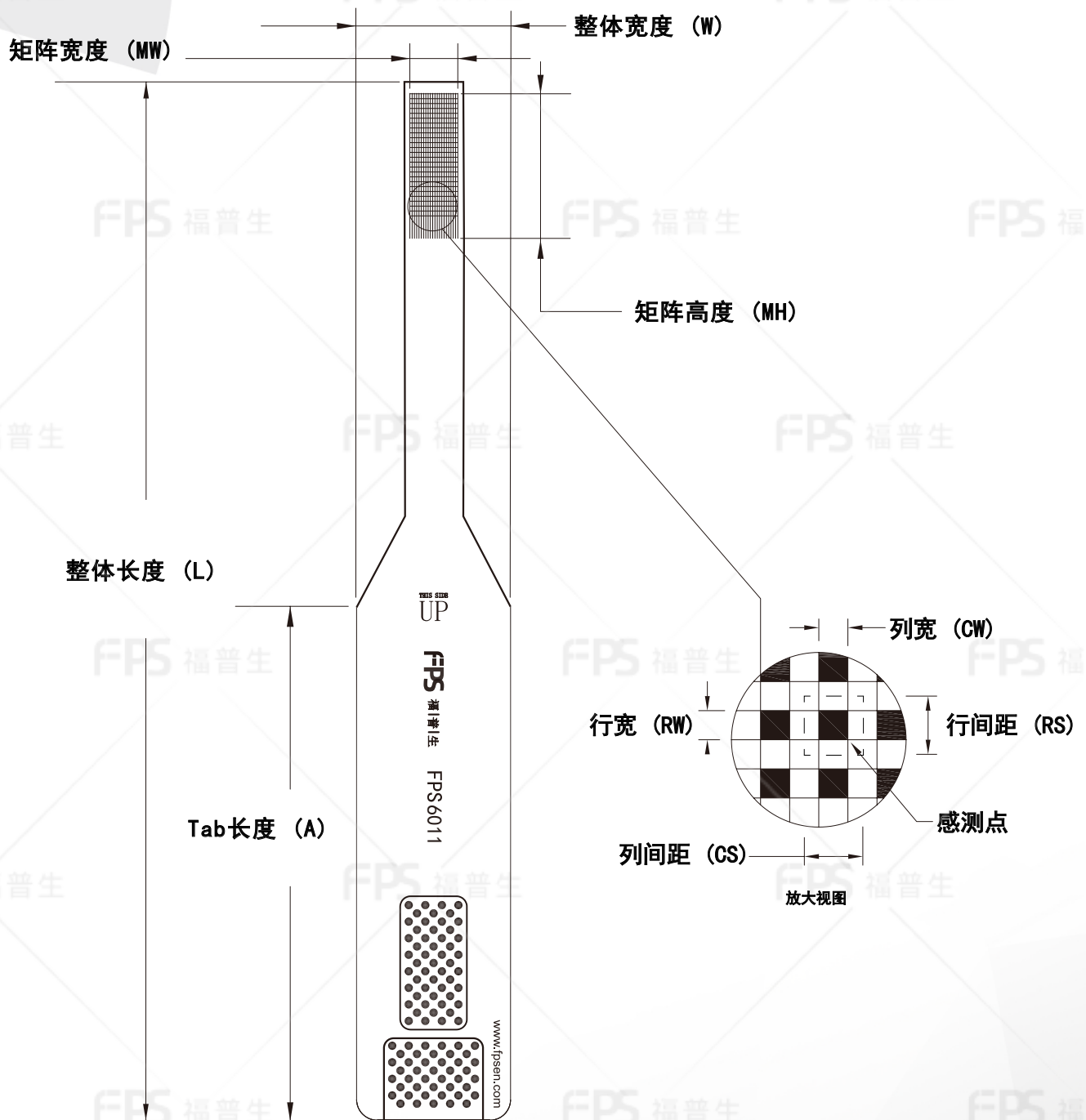
外形尺寸
