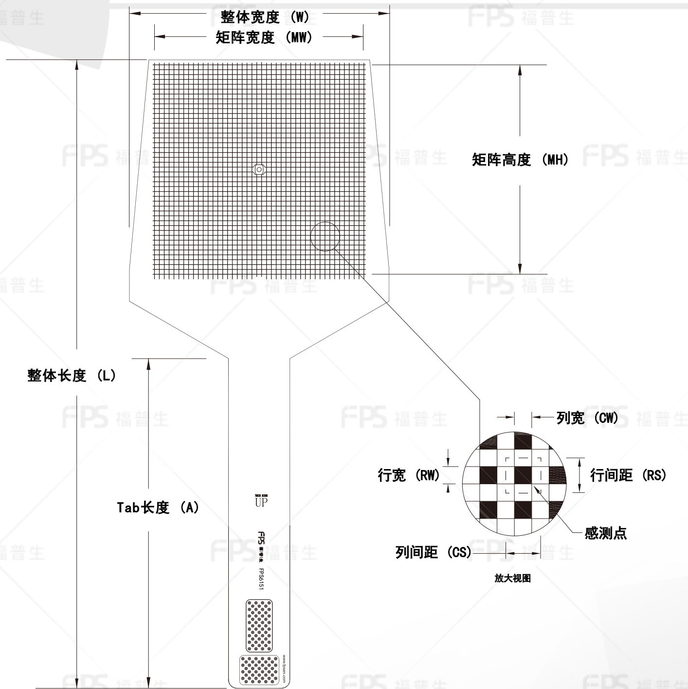
外形尺寸
