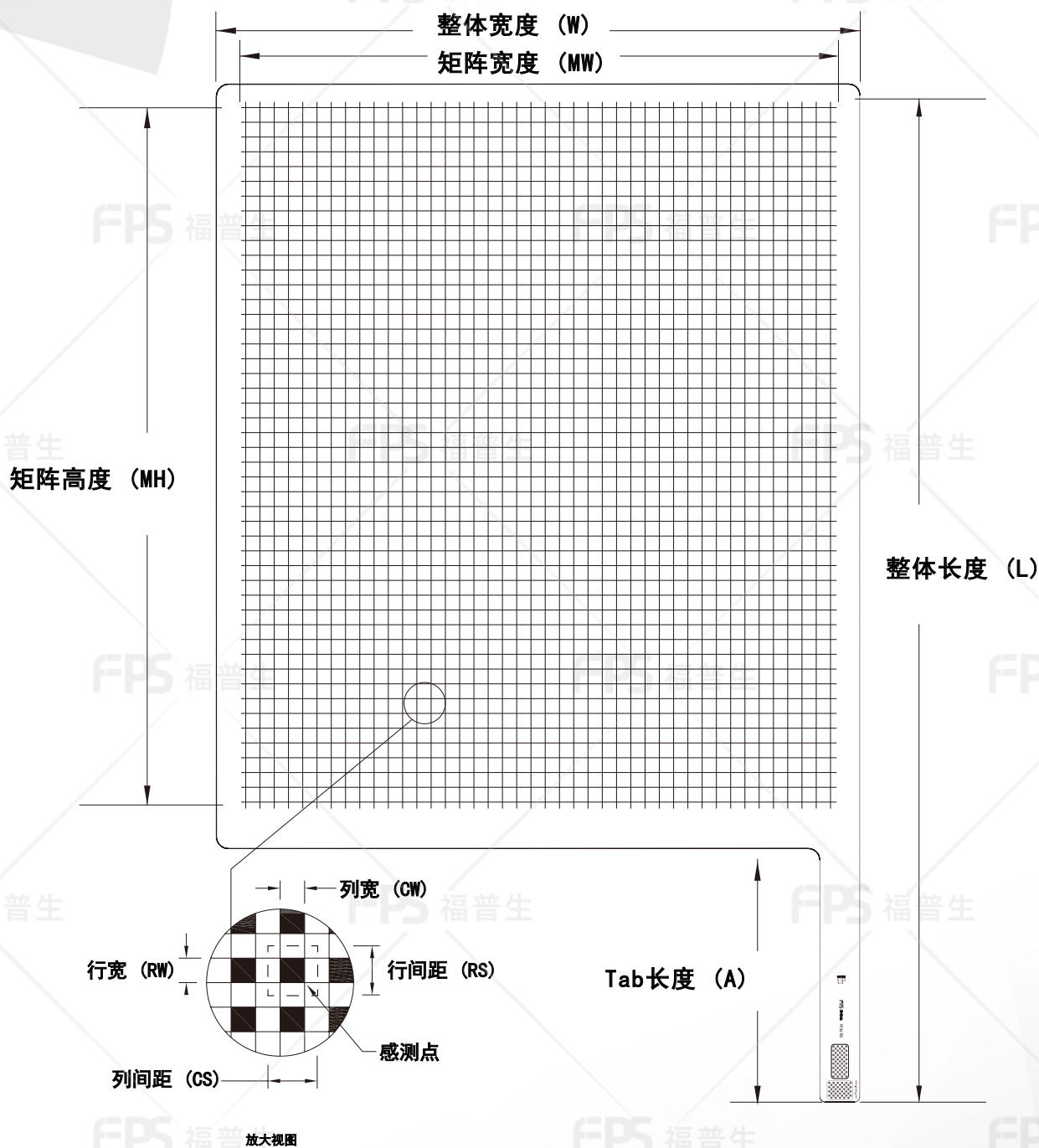
外形尺寸
