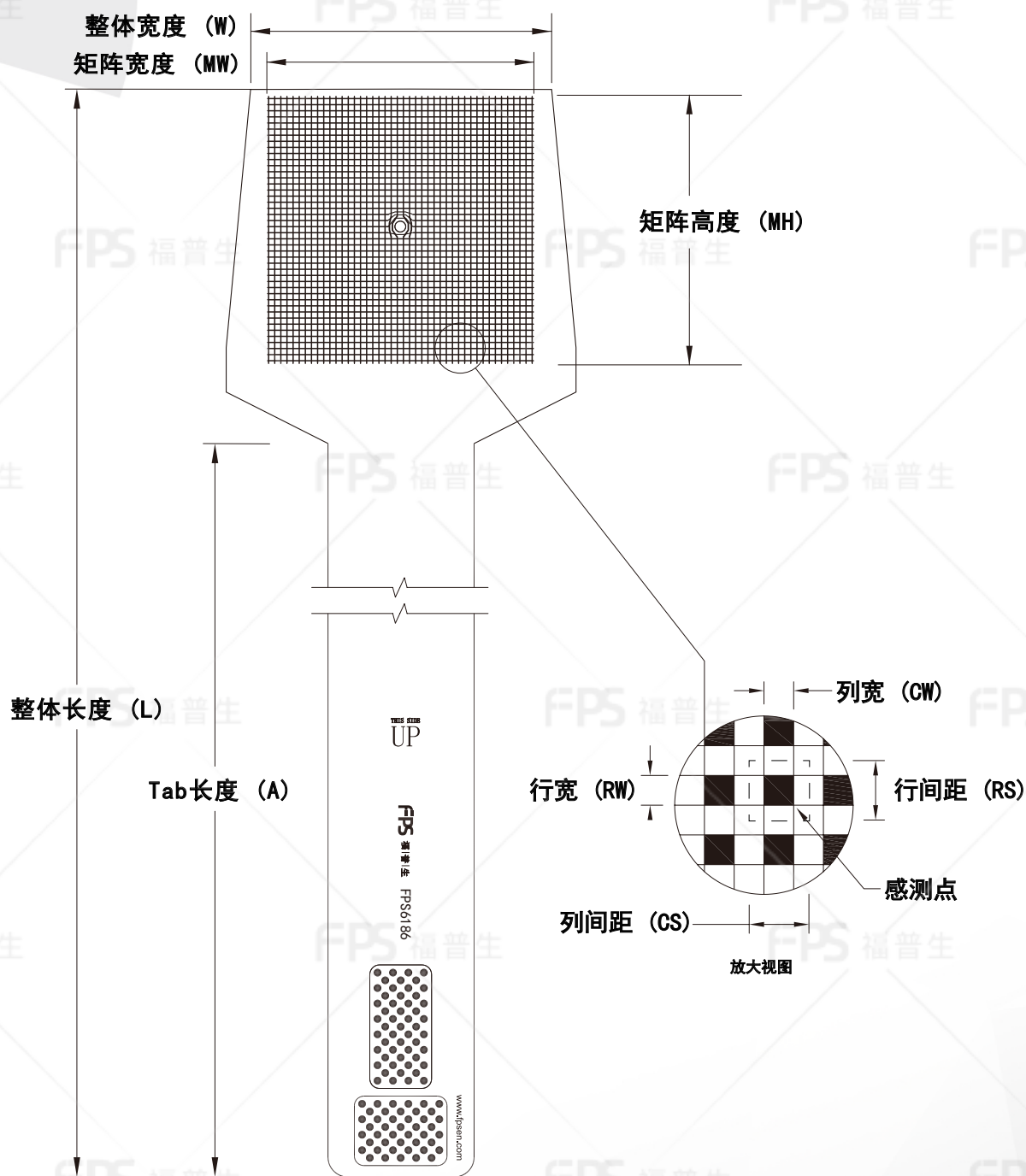
外形尺寸
