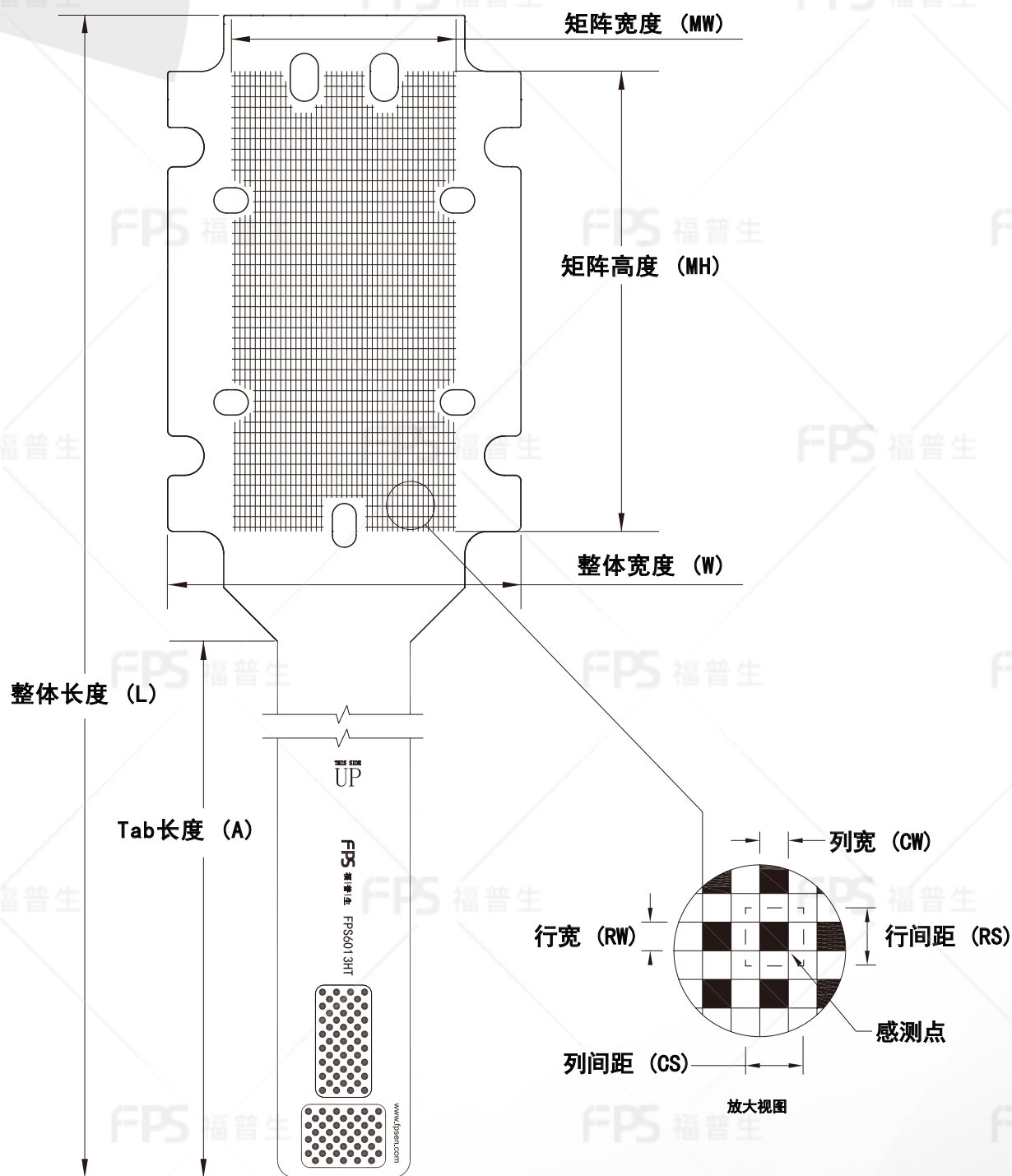
外形尺寸
