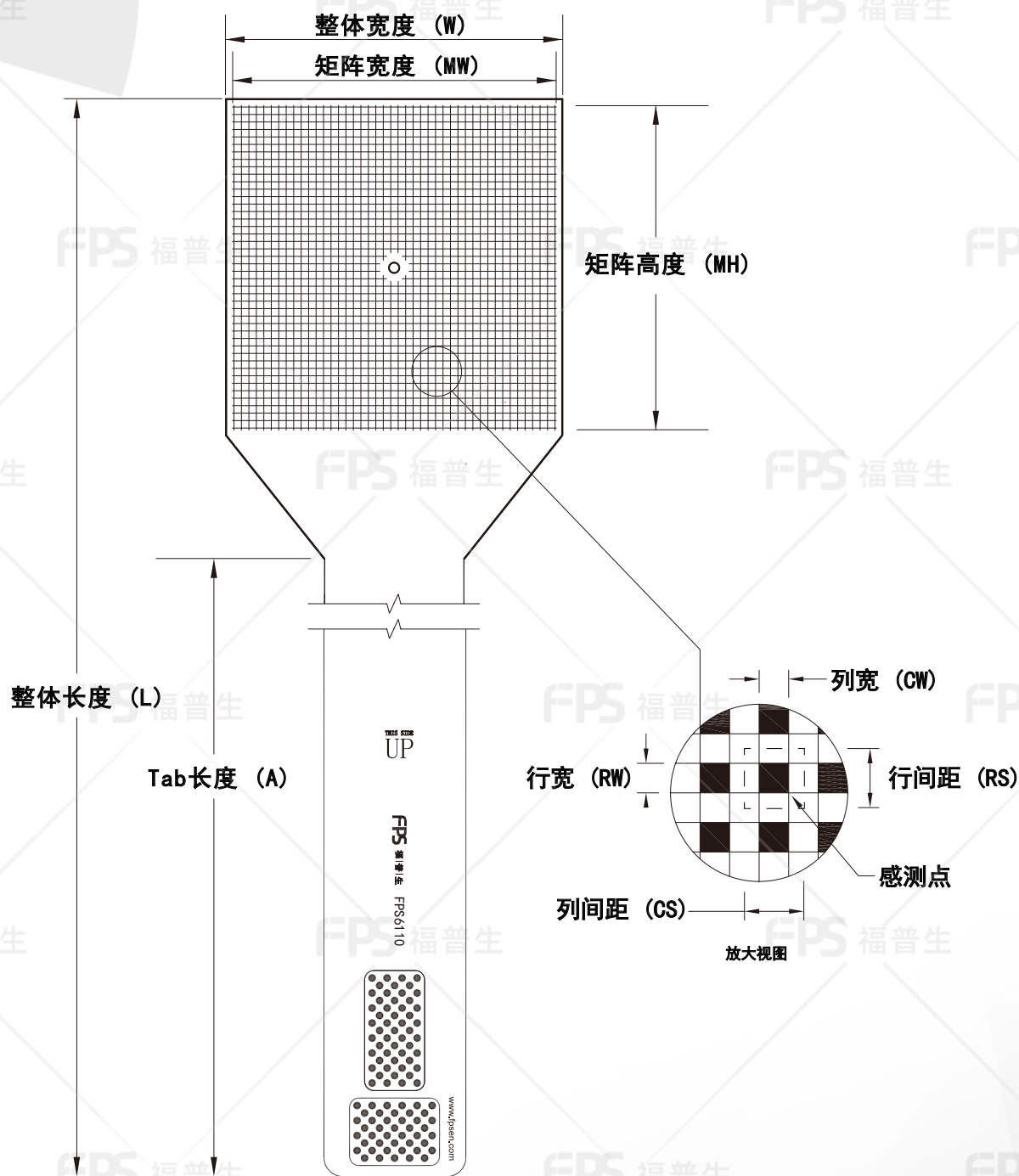
外形尺寸
